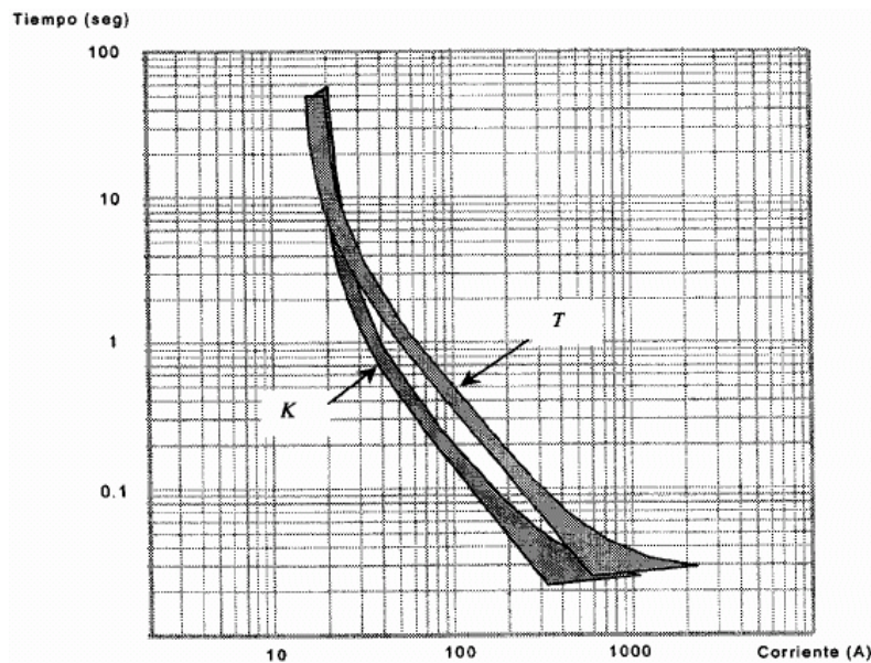
Figura B.10.- Diferencia de respuesta para fusibles tipo K y T.
