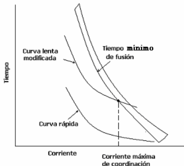
Figura. 4.7.- Coordinación fusible-restaurador.
