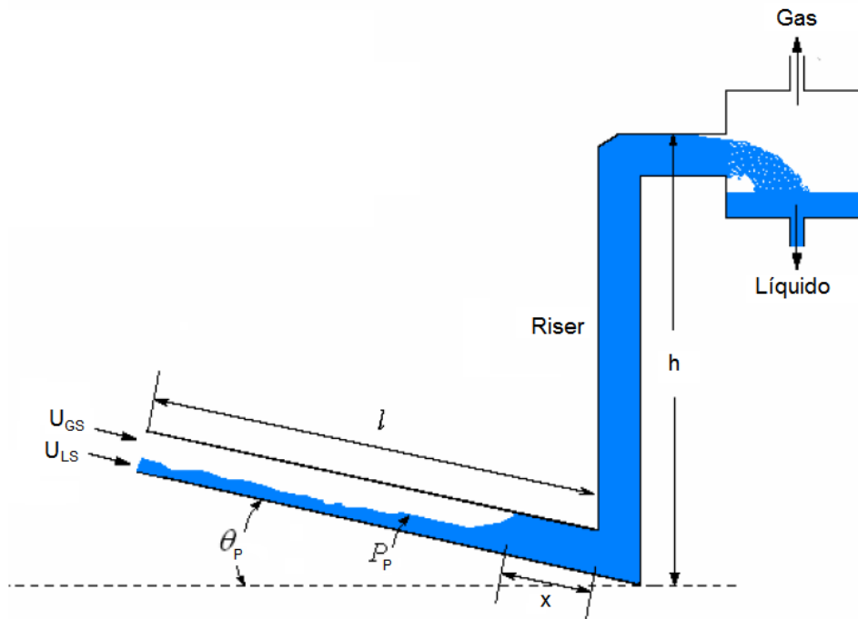
Figura 1.12 Segunda etapa de formación del flujo slug severo.
