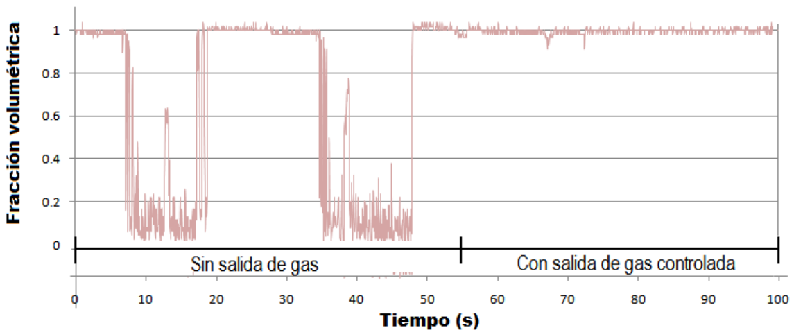
Figura 4.22 Fracción volumétrica durante el slug severo y controlando la salida de gas
