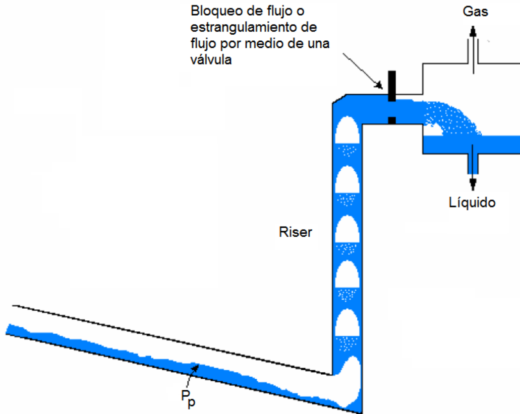
Figura 1.15 Técnica de bloqueo o de estrangulamiento de flujo.
