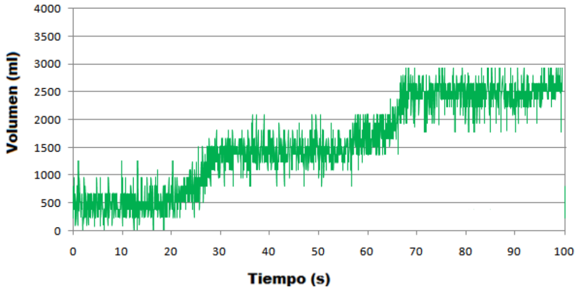
Figura 3.6 Gráfica de de volumen medido con TP5 para el separador de fases
