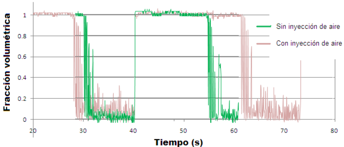
Figura 4.18 Fracción volumétrica inyección de aire en el codo.
