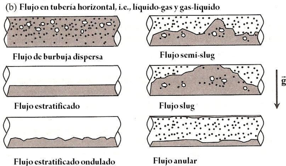
Figura 1.6 Patrones de flujo para tuberías ligeramente inclinadas
