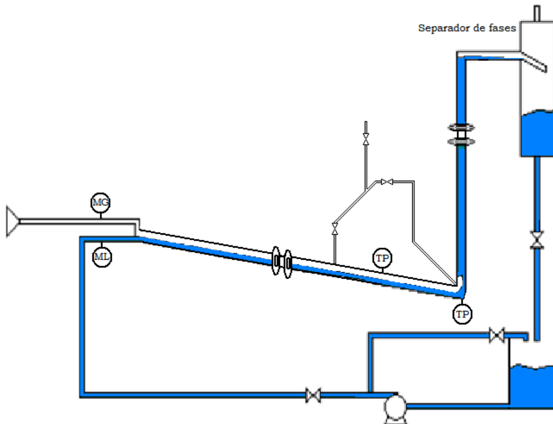
Figura 2.12 Diagrama experimental 2 sistema de inyección de aire
