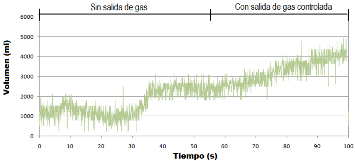
Figura 4.23 Volumen durante el slug severo y controlando la salida de gas.
