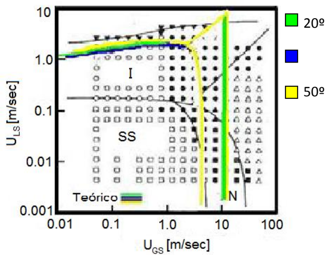
Figura 1.5 Patrones de flujo con una tubería en inclinación ascendente
