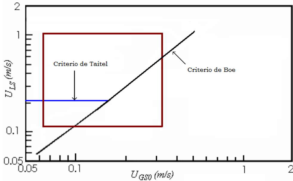
Figura 2.3 Criterio de Boe y Taitel sobre la existencia del slug severo.
