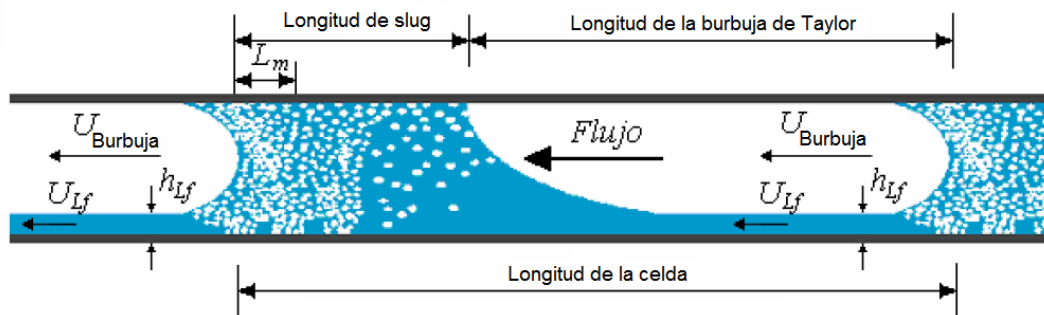
Figura 1.2 Celda de flujo slug de una tubería horizontal
