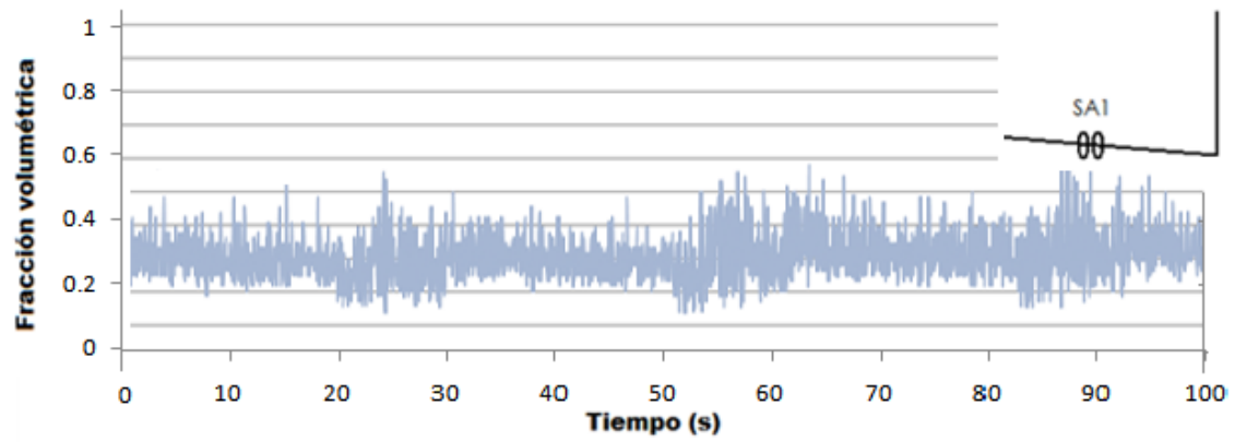
Figura 3.4 Fracción volumétrica captada por las sondas SA1 y SA2
