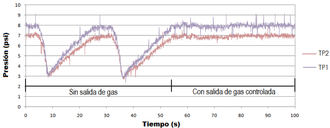
Figura 4.20 Presiones durante el slug severo y controlando la salida de gas
