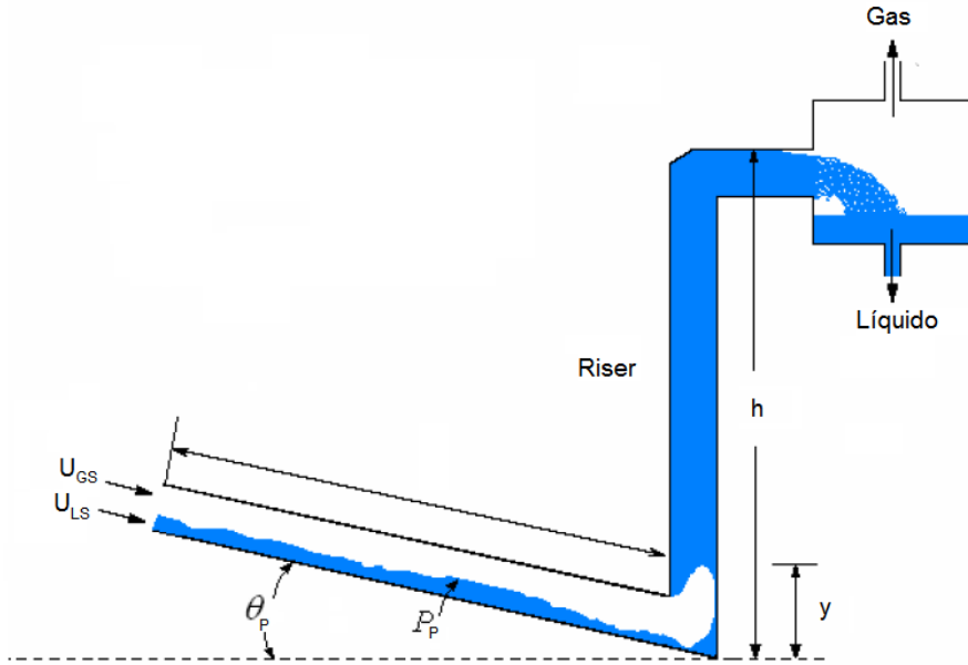
Figura 1.13 Tercera etapa de la formación del slug severo.
