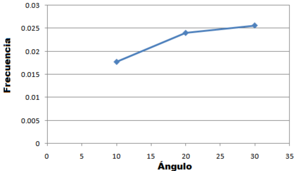
Figura 4.11 Variación de la frecuencia con respecto al ángulo del codo para U_{SL} = 0.066 \text{ m/s} U_{SG} = 0.066 \text{ m/s}
