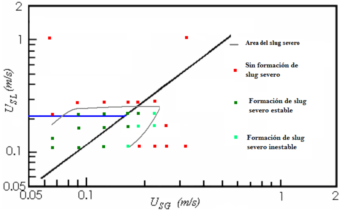
Figura 3.8 Resultados de los experimentos realizados para la geometría ( L1=4m , L2=3m , \theta=30^\circ )
