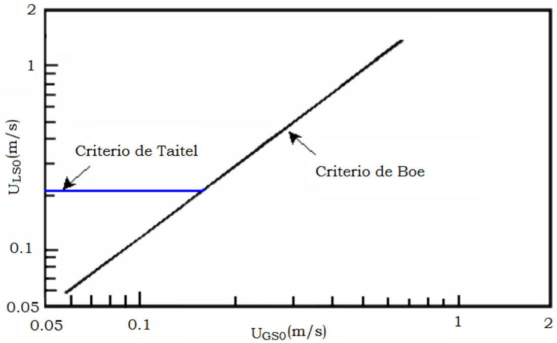
Figura 1.18 Criterios de Boe y Taitel en grafico de velocidades superficiales de gas y líquido.
