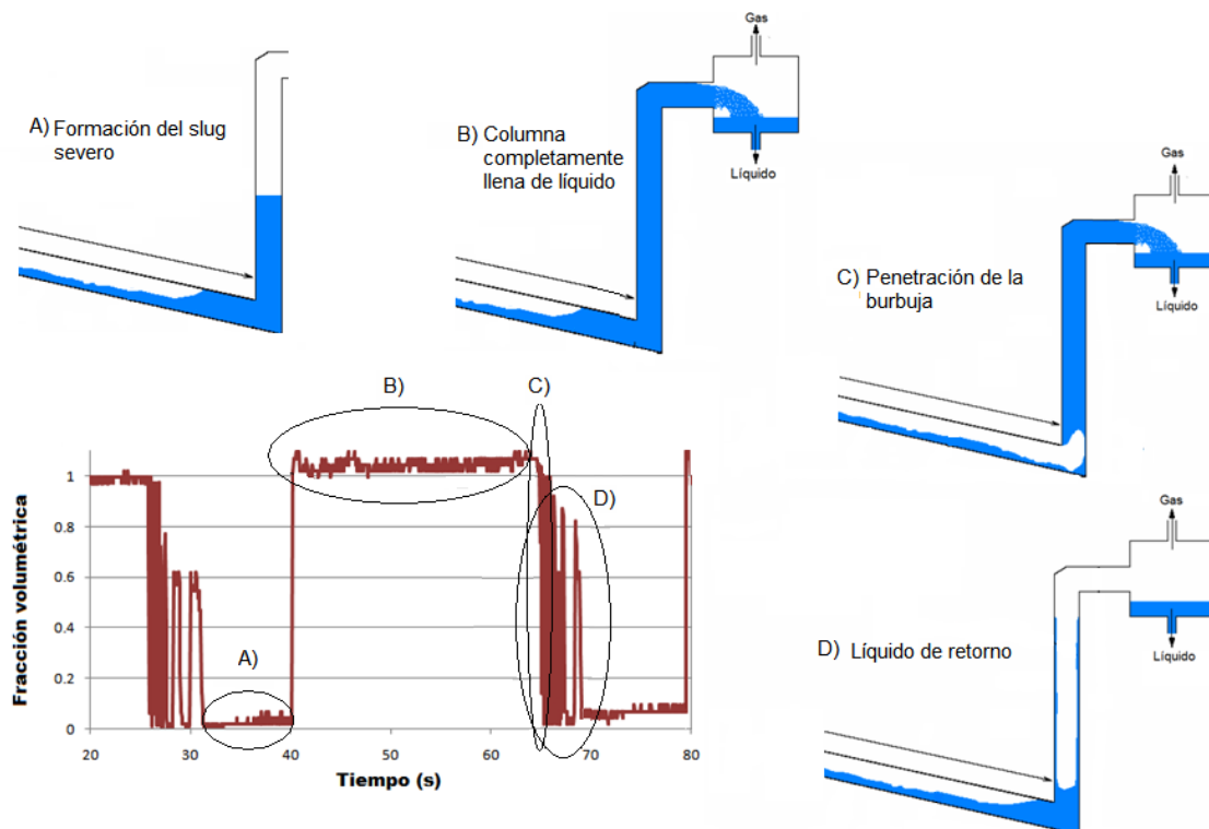
Figura 4.9 Etapas de formación del slug para U_{SL} = 0.066 \text{ m/s} , U_{SG} = 0.066 \text{ m/s}
