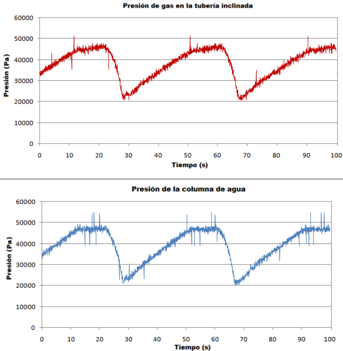
Figura 3.3 Gráficas de presión para los transductores de presión
