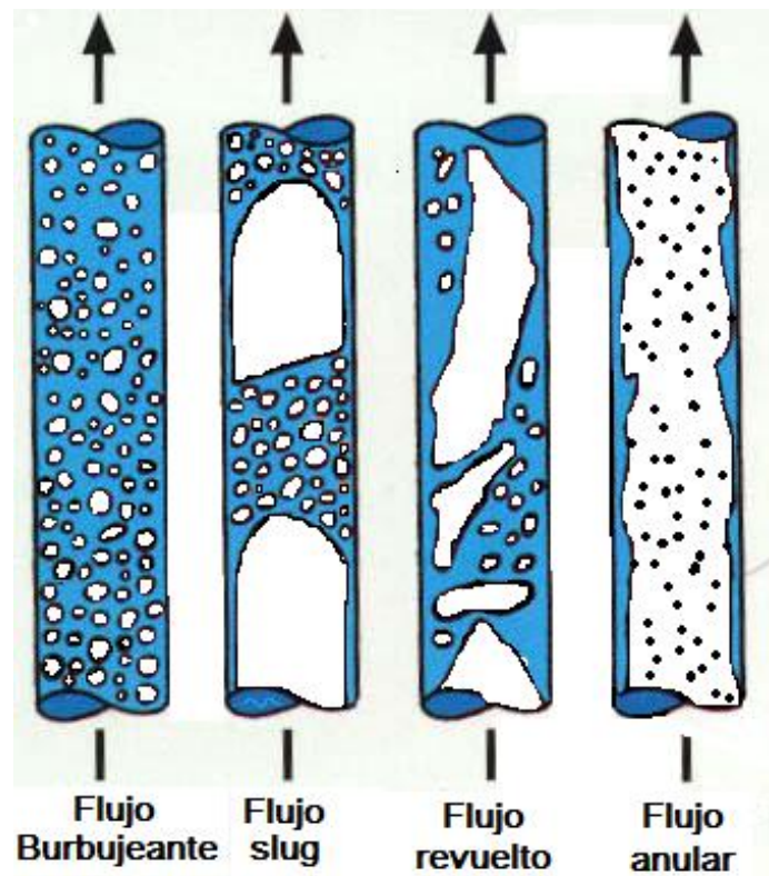
Figura 1.8 Patrones de flujo para tuberías verticales.
