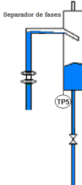
Figura 4.6 Medidor de presión calibrado para medir volumen.
