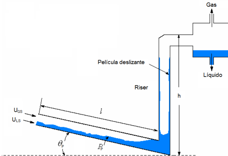
Figura 1.14 Cuarta etapa de la formación del slug severo.
