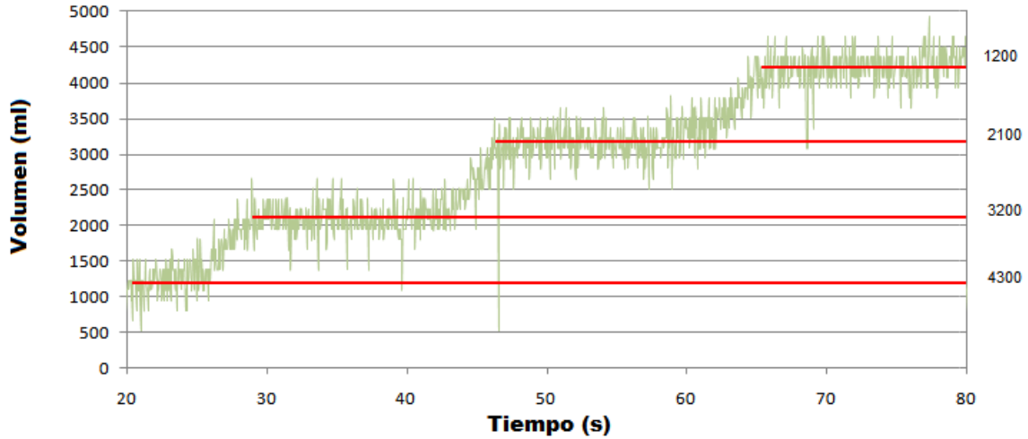
Figura 4.7 Volumen en el separador para U_{SL} = 0.132 \text{ m/s} y U_{SG} = 0.132 \text{ m/s}
