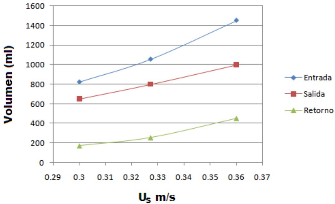
Figura 4.8 Resultados de volúmenes en el entrada al riser, de salida al separador y de retorno.
