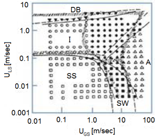
Figura 1.3 Patrones de flujo para una tubería horizontal de 25mm de diámetro, utilizando fluidos de trabajo agua-aire a condiciones atmosféricas.
