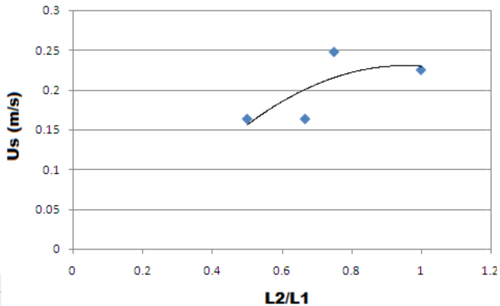
Figura 4.16 Variación de la velocidad del slug con respecto a la longitud de los tramos
