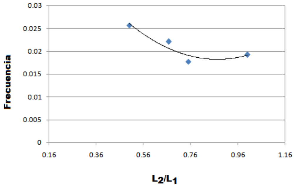
Figura 4.15 Variación de la frecuencia del slug con respecto a la longitud de los tramos
