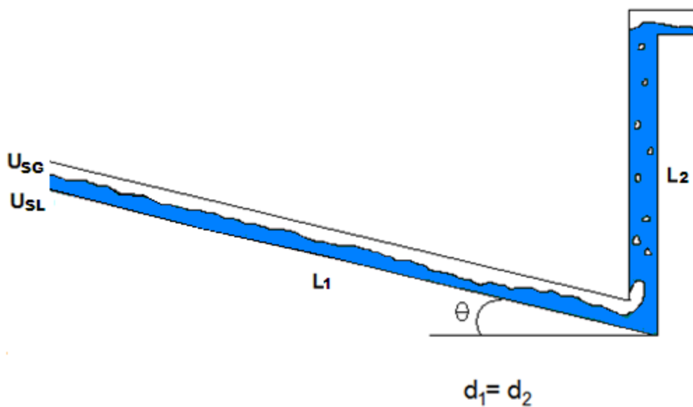
Figura 2.1 Variables geométricas y de proceso a considerar.
