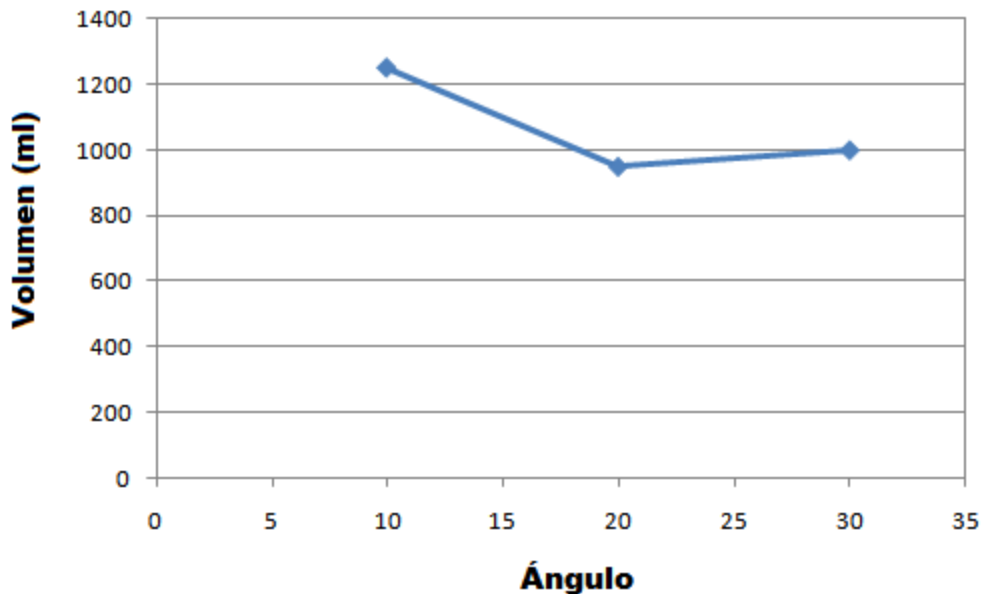
Figura 4.13 Variación del volumen del separador con respecto al ángulo del codo para U_{SL} = 0.066 \text{ m/s} U_{SG} = 0.066 \text{ m/s}
