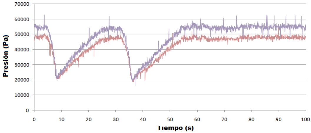
Figura B.2 Presiones TP1 y TP2
