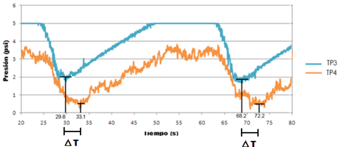
Figura 4.4 Gráfica presión de dos transductores separados 90 cm.
