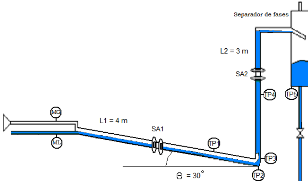
Figura 4.1 Geometría de la instalación experimental.
