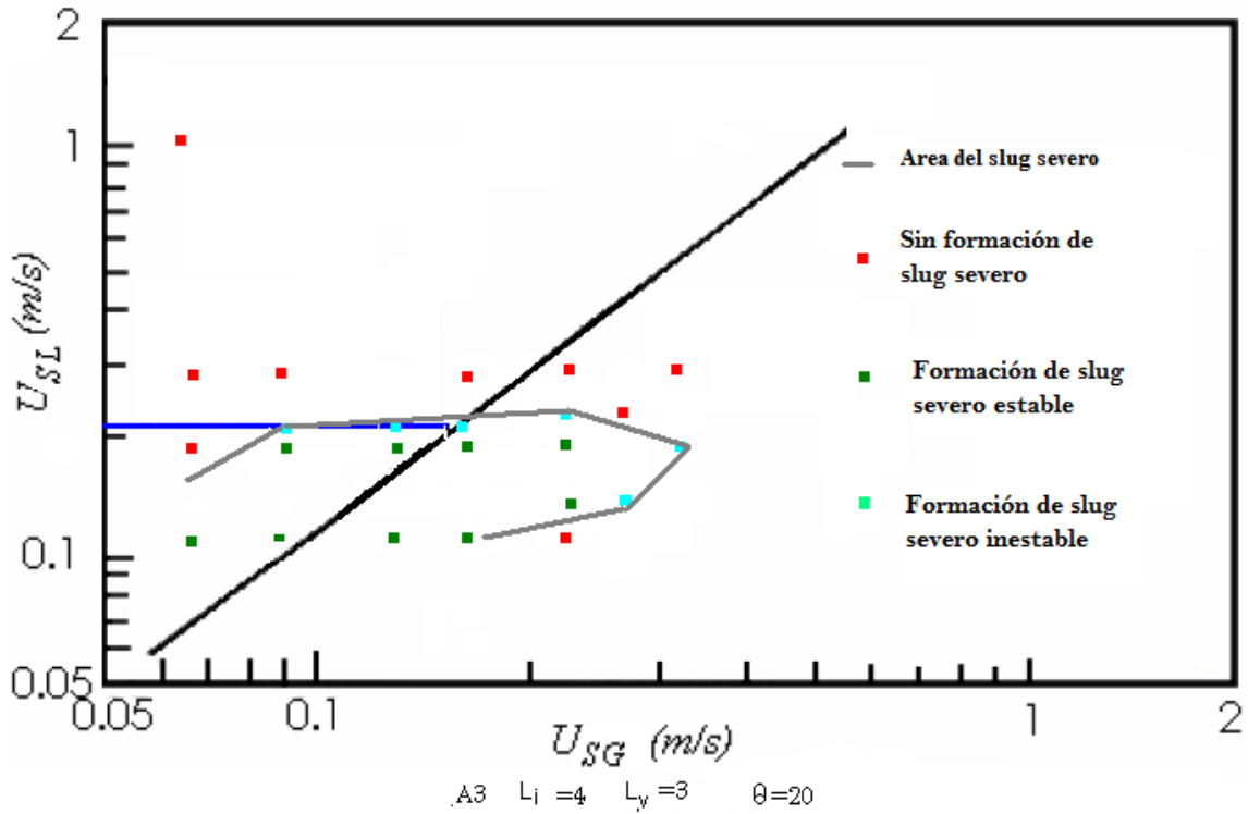
Figura A.3 Corridas experimentales de la geometría A3
