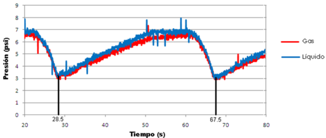
Figura 4.2 Frecuencia del slug severo para el experimento
