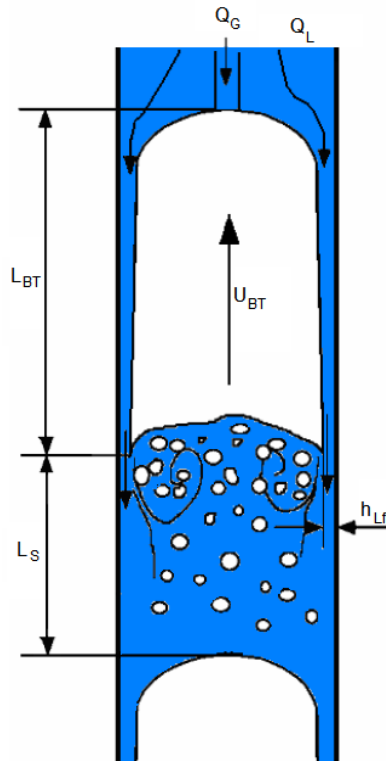
Figura 1.9 Flujo slug en una tubería vertical.
