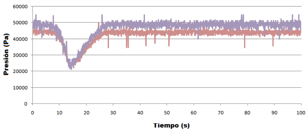
Figura B.17 Presiones TP1 y TP2
