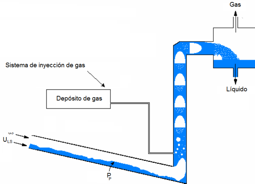
Figura 1.16 Técnica de inyección de gas (gas-lift).
