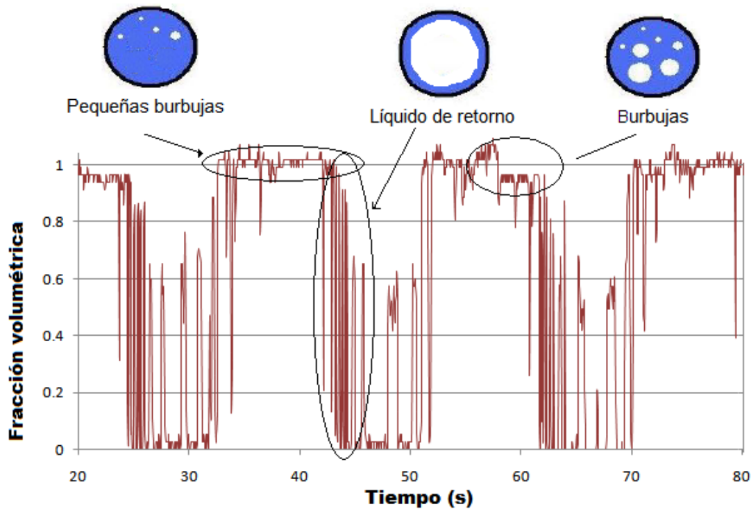
Figura 4.10 Penetración de burbujas durante el slug severo U_{SL} = 0.132 \text{ m/s} U_{SG} = 0.132 \text{ m/s}
