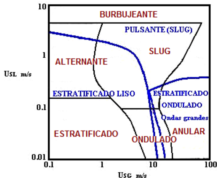
Figura 1.7 Mapa de régimen de flujo (línea azul), tubería de 2.5 cm con 10° de inclinación descendente. Agua y aire como fluidos de trabajo a presión atmosférica. Comparación contra la carta de patrón de flujo horizontal de Mandhane.
