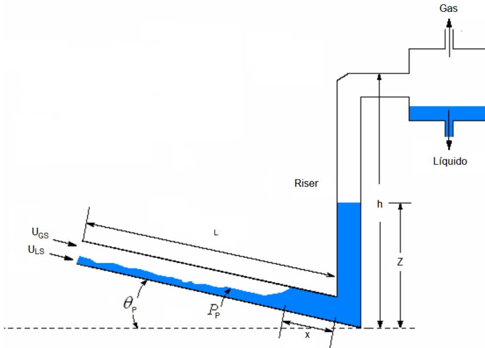
Figura. 1.11 Primera etapa de formación del flujo slug severo.
