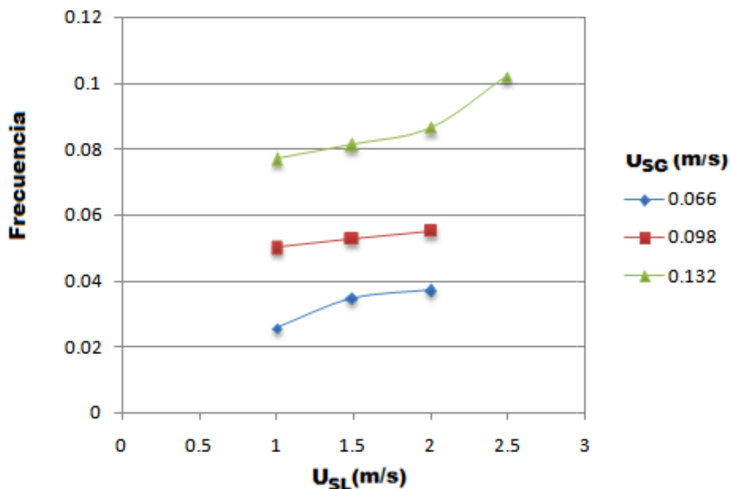
Figura 4.3 Frecuencia para U_{SL} = constante
