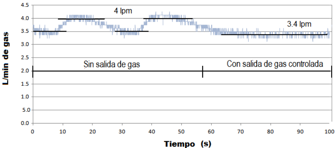
Figura 4.24 Flujo de gas a la entrada del sistema
