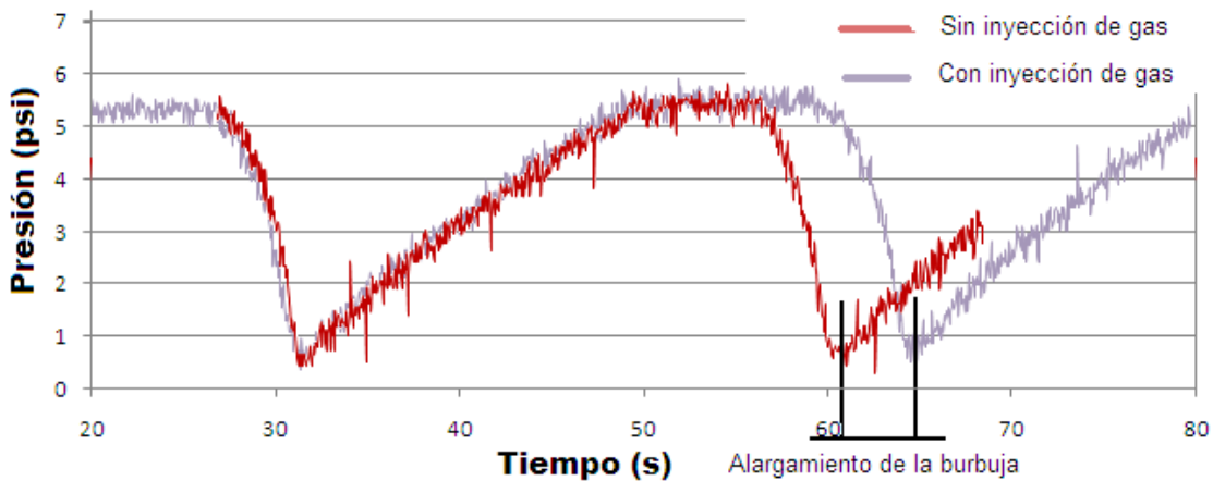
Figura 4.17 Presión para TP2 inyección de aire en el codo.
