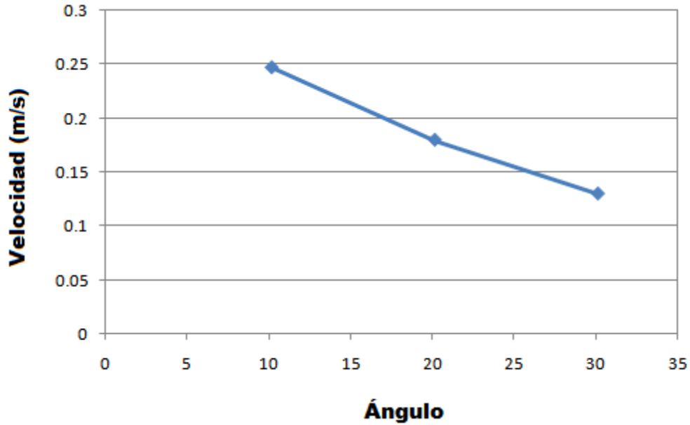
Figura 4.12 Variación de la velocidad del slug con respecto al ángulo del codo para U_{SL} = 0.066 \text{ m/s} U_{SG} = 0.066 \text{ m/s}
