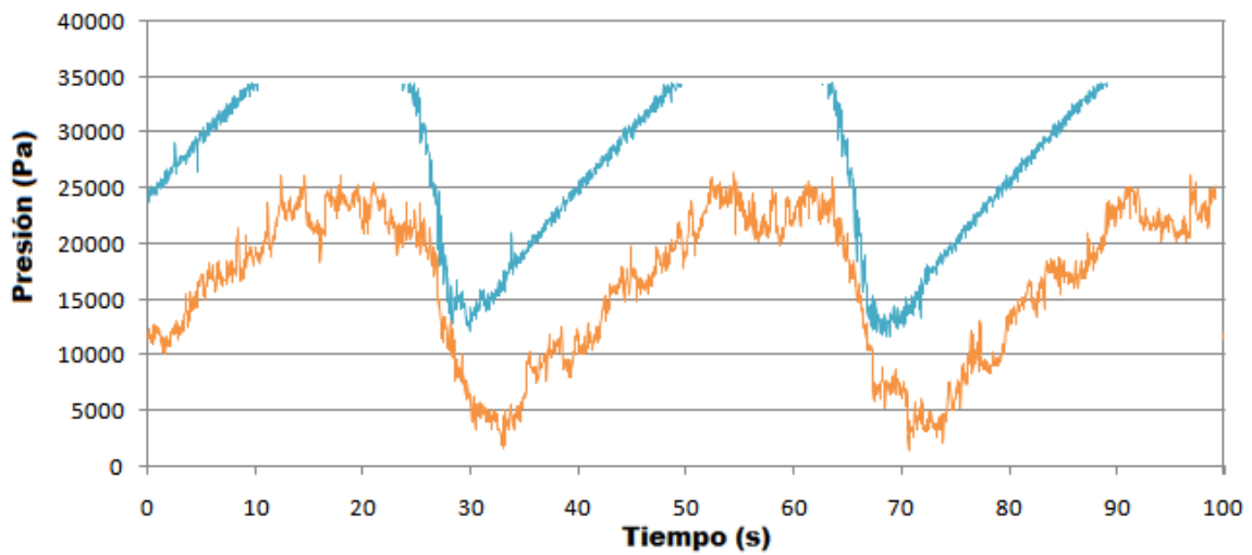
Figura 3.5 Gráfica de TP_3 y TP_4 para la medición de presión
