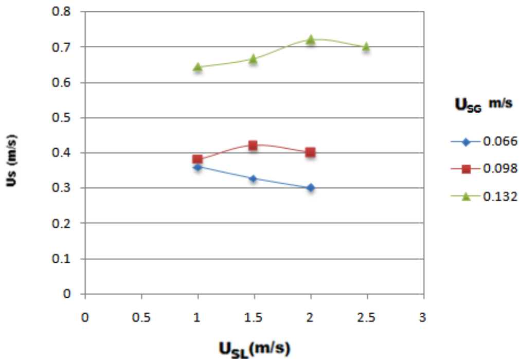
Figura 4.5 Velocidad de salida del slug severo.
