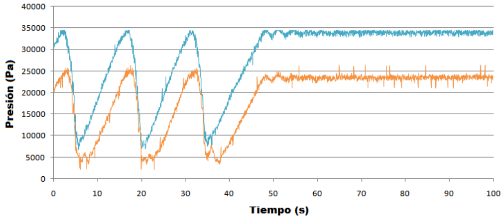
Figura B.10 Volumen de llegada al separador de fases
