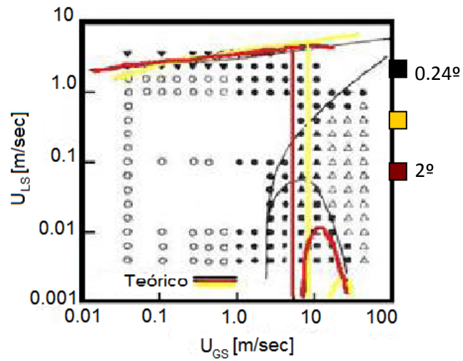
Figura 1.4 Patrones de flujo con una tubería en inclinación descendente.
