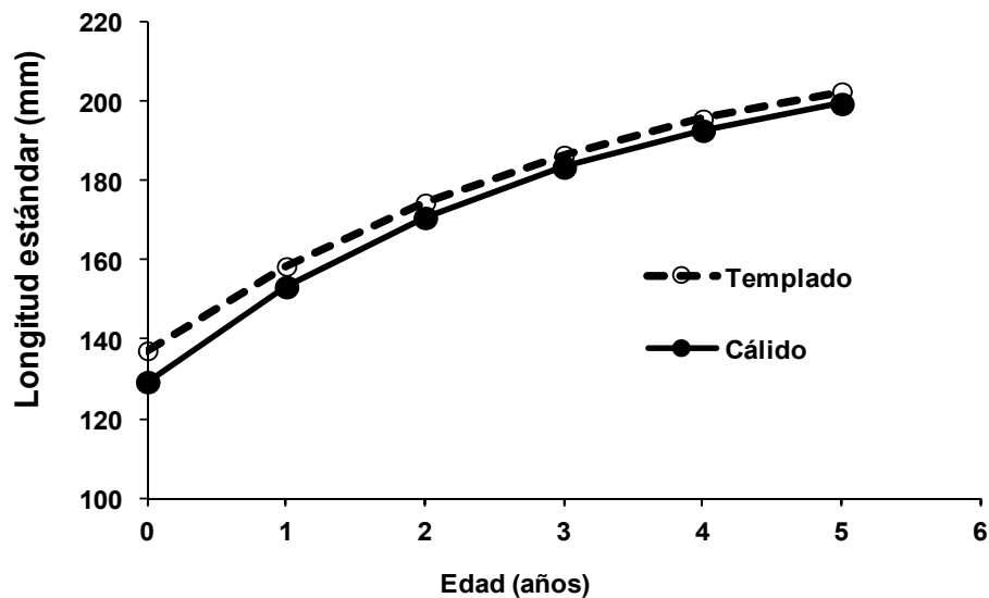
Figura 11. Curvas de crecimiento individual de la sardina del Pacífico por stock durante en Bahía Magdalena, durante 1982 a 2009. Stock cálido (línea sólida) y el templado (línea punteada).
