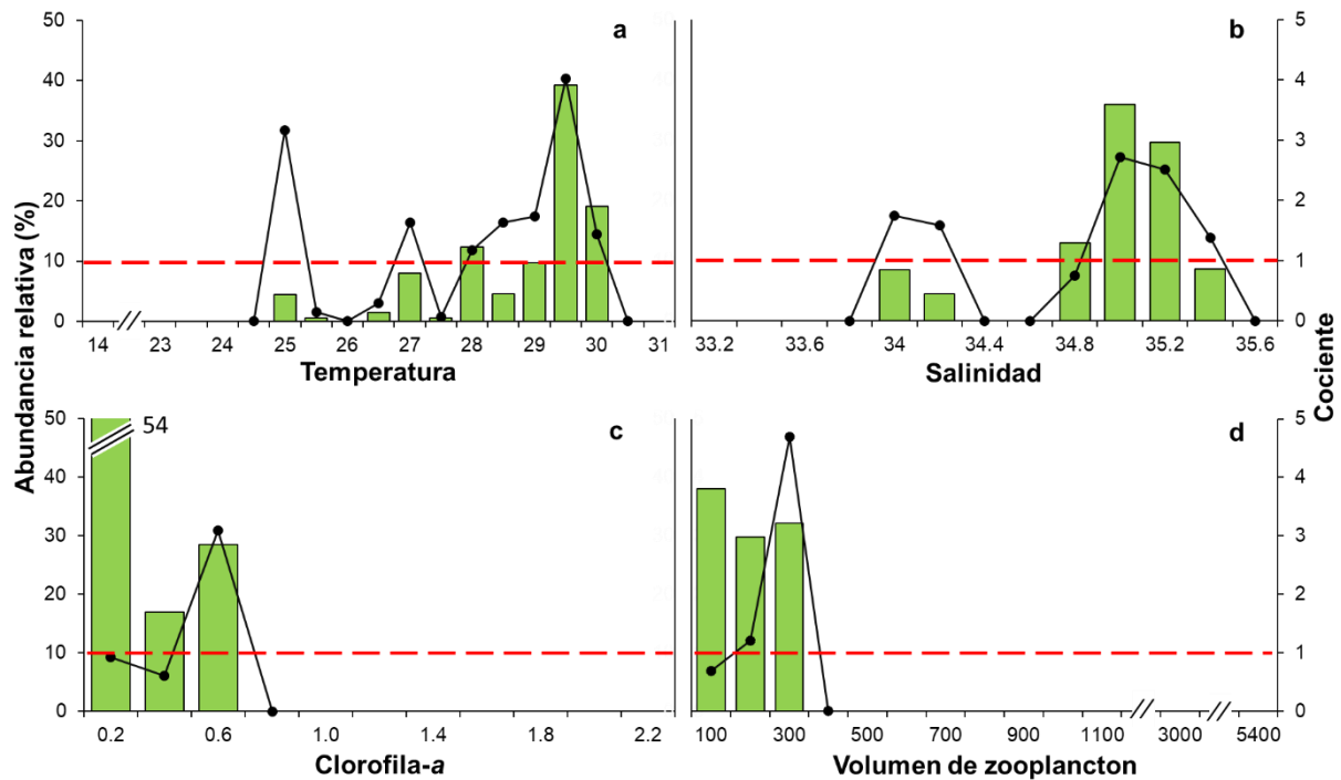
Figura 19. Curvas de cocientes de las variables analizadas para el Complejo SD. a) temperatura (°C), b) salinidad, c) concentración de clorofila-a (mg/m 3 ) y d) volumen de zooplancton (ml/1000 m 3 ). La línea roja punteada representa cocientes \geq 1 , que indican una selección significativa. Las barras indican la abundancia relativa de PL. Las líneas con punto indican los cocientes.
