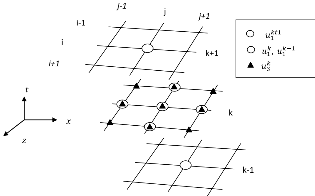
Figura 3.7. Esquema de discretización para el caso P-SV en 2D mediante diferencias finitas. Donde se emplean desplazamientos tanto horizontales u_1 , como verticales u_3 , en el tiempo k .
