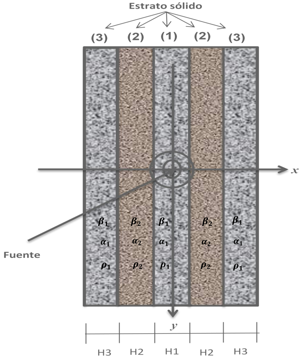
Figura 4.4. Sistema de estratos sólidos, con diferentes propiedades mecánicas.
