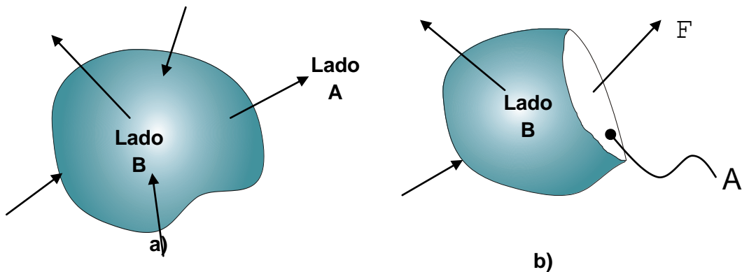
Fig. 2.1 a) Cuerpo sometido a un estado de fuerzas, b) Diagrama de cuerpo libre de la porción B
