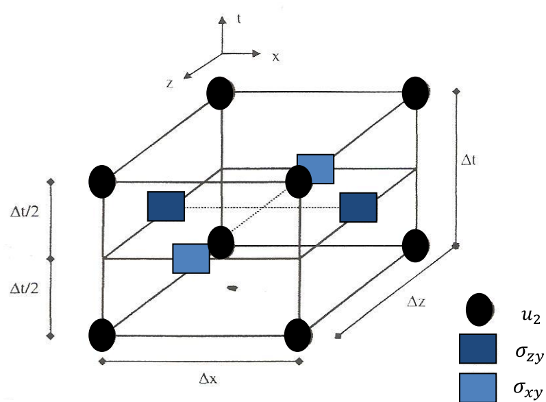
Figura 3.6. Discretización del medio con una malla alternada para el problema SH.
