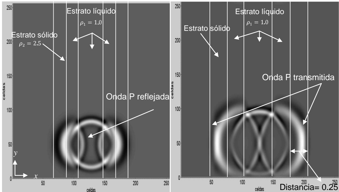
Figura 4.33. Propagación de ondas P transmitida y reflejada en un multi-estrato líquido-sólido, en un instante de un tiempo de 0.00036 y 0.00044 segundos.
