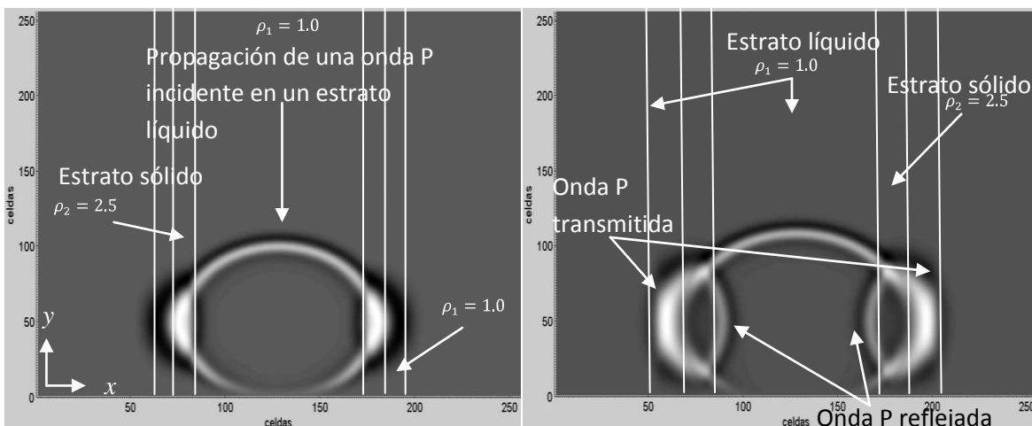
Figura 4.23, propagación de una onda P en un medio líquido confinados en dos medios solidos, en una instantánea de un tiempo de 0.00047 y 0.00052 segundos.
