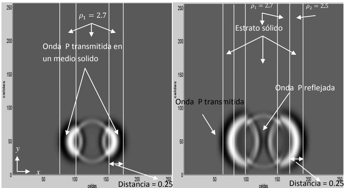
Figura 4.16. Propagación de ondas P transmitidas y reflejadas en un medio sólido, en una instantánea de tiempo de 0.00033 y 0.00038 segundos.
