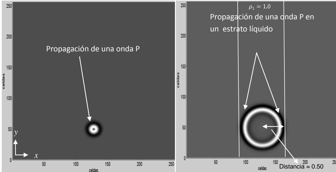
Figura 4.21. Propagación de una onda P en un estrato líquido, en una instantánea de un tiempo de 0.00016 y 0.00033 segundos.
