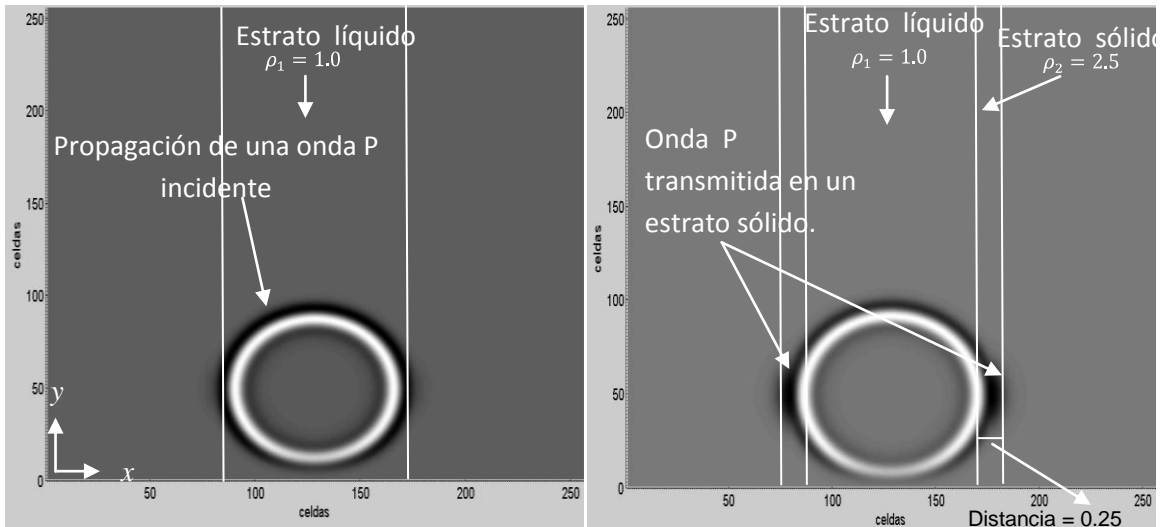
Figura 4.22. Propagación de una onda P transmitida en un estrato sólido, en una instantánea de un tiempo 0.00038 y 0.00041 segundos.
