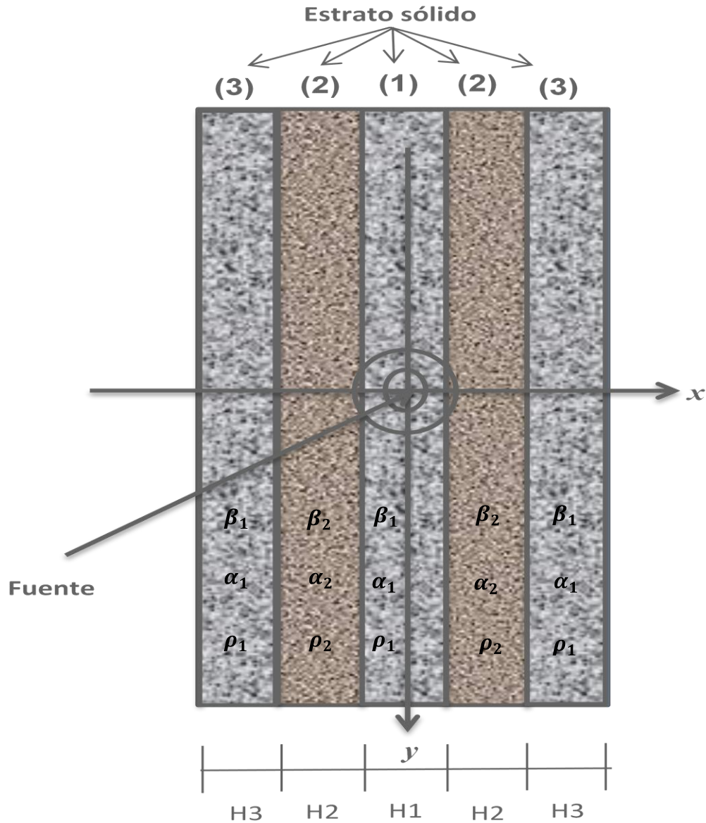
Figura 1.1. Sistema de múltiples estratos sólidos, con diferentes propiedades mecánicas.
