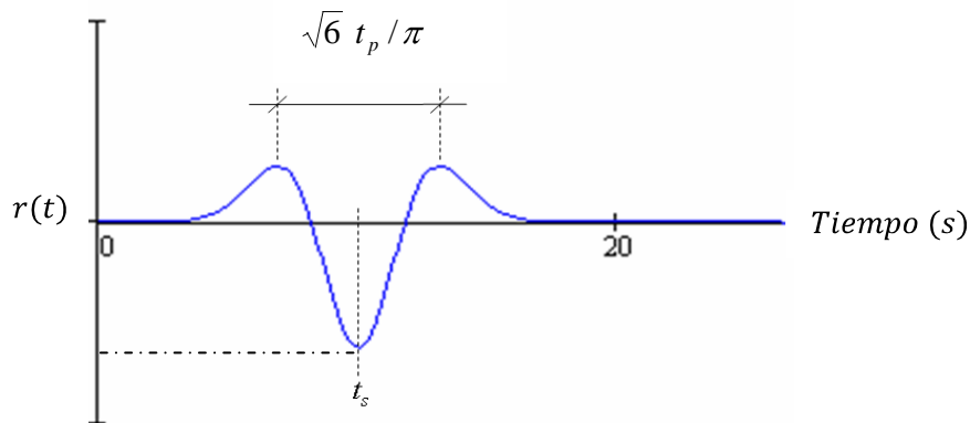
Fig. 3.1. Representación del Pulso de Ricker en el dominio del tiempo.
