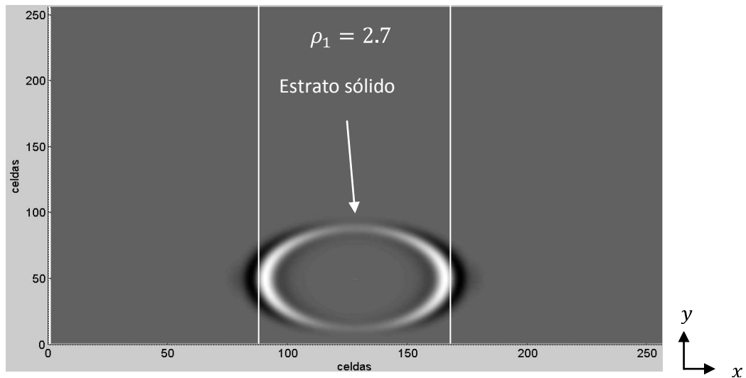
Figura 4.7. Propagación de una onda P, en un instante de un tiempo de 0.00038 segundos.
