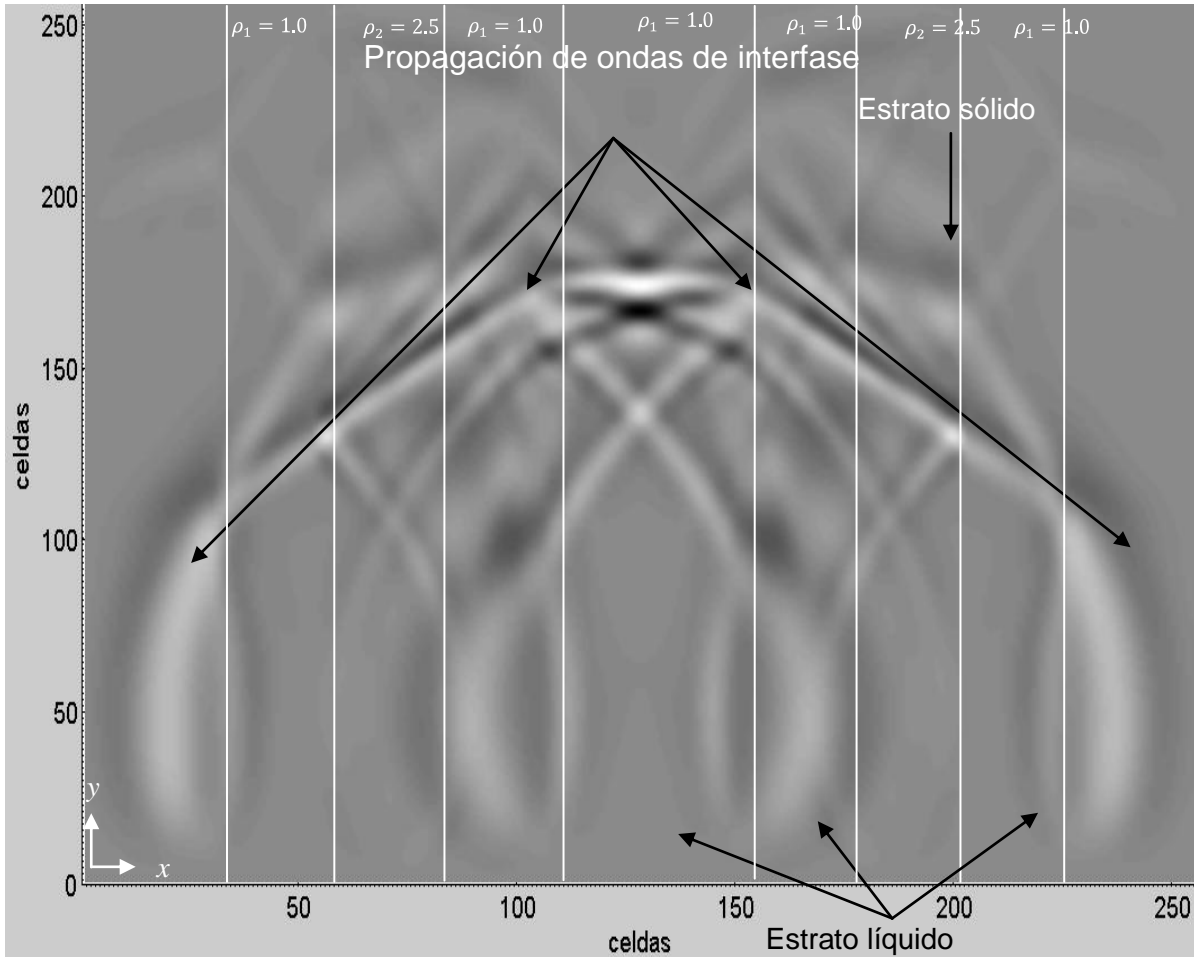
Figura 4.37. Propagación de las ondas de Interfase en un multi-estrato líquido-sólido, en un instante de un tiempo de 0.00097 segundos.
