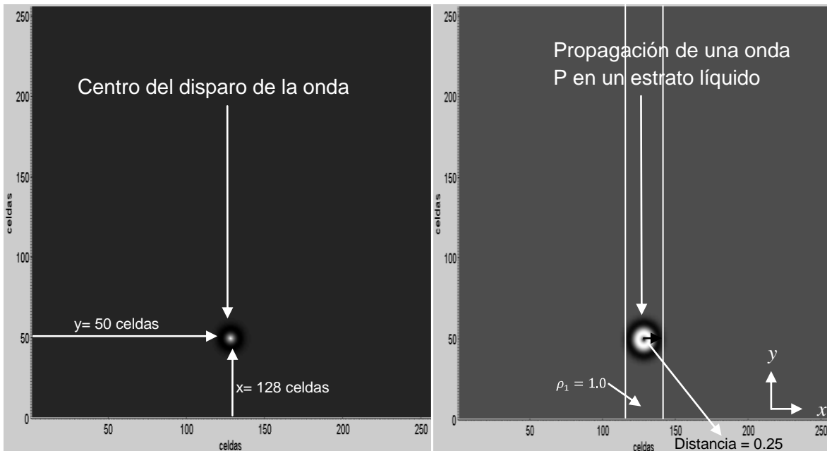
Figura 4.30. Propagación de una onda P en un estrato líquido, en una instantánea de un tiempo 0.00013 y 0.00016 segundos.
