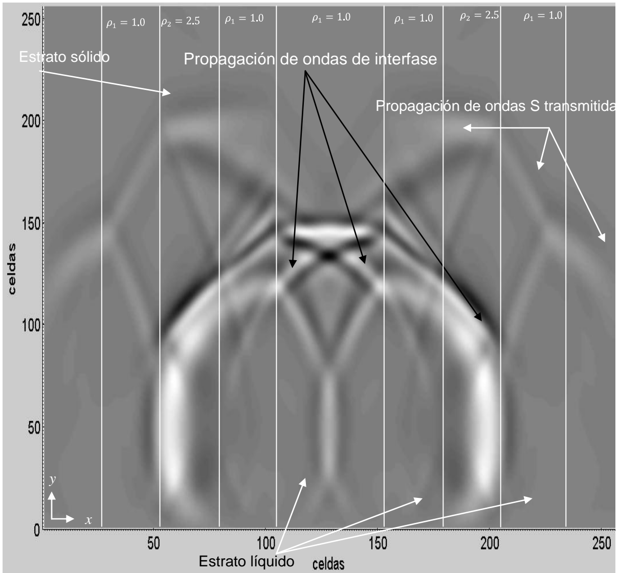
Figura 4.36. Propagación de ondas de Interfase en un multi-estrato líquido-sólido, en un instante de un tiempo de 0.00077 segundos.
