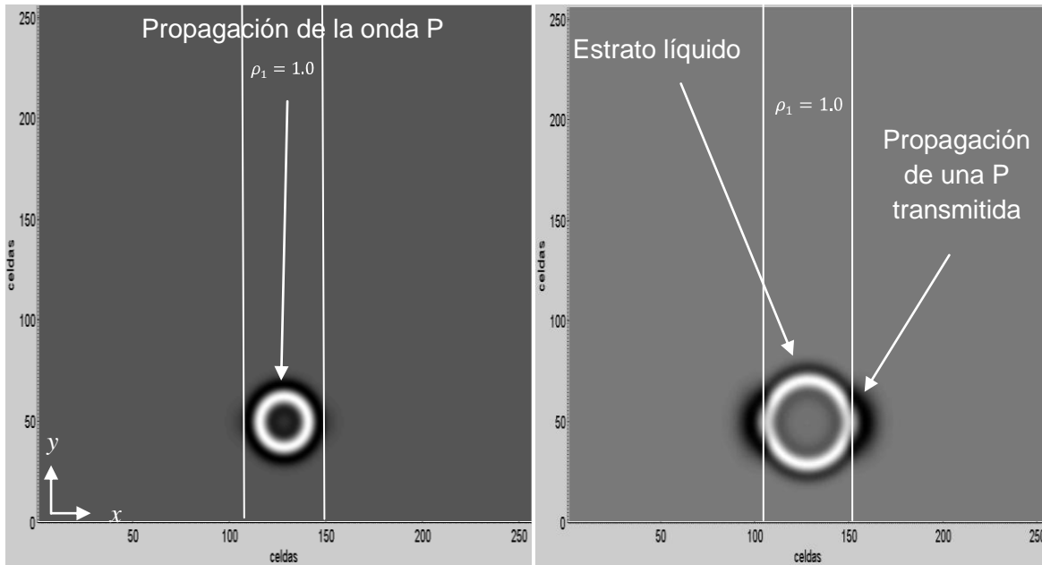
Figura 4.31. Propagación de una onda P transmitida en un estrato líquido confinado a un medio sólido, en una instantánea de un tiempo de 0.00022 y 0.00027 segundos.
