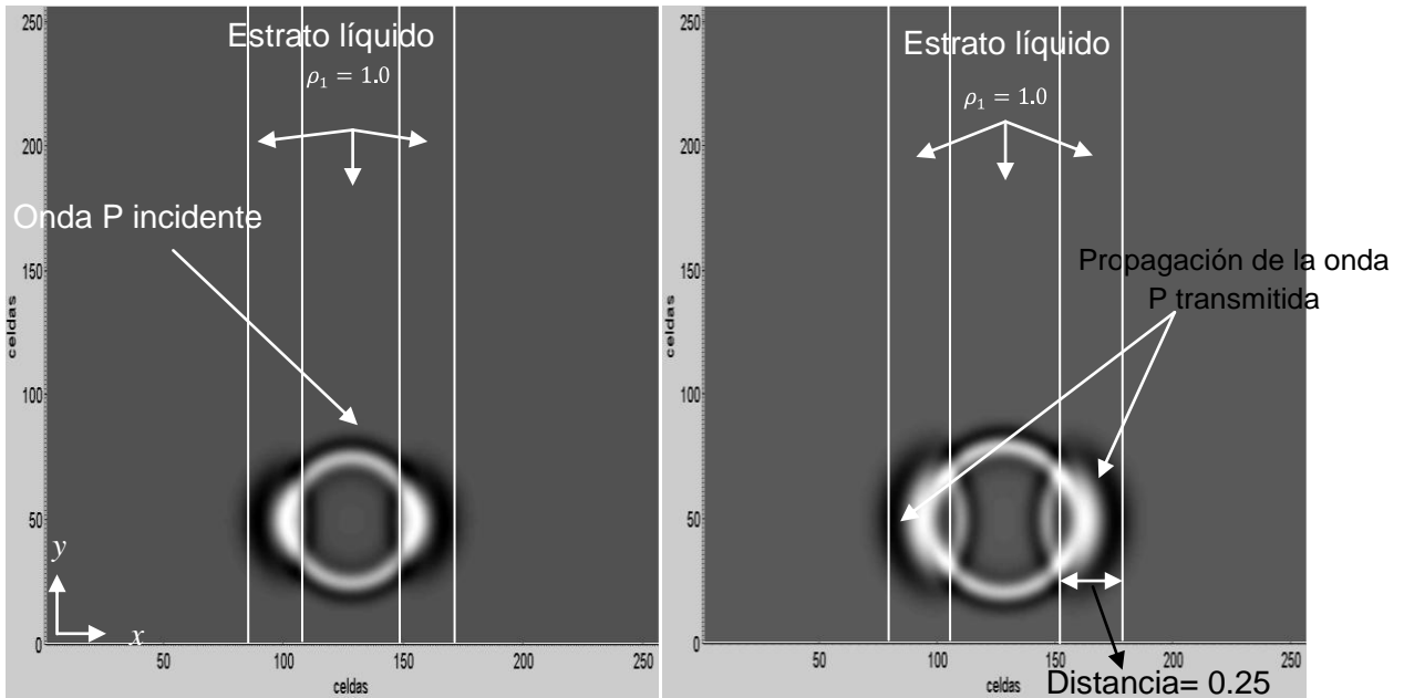
Figura 4.32. Propagación de una onda P incidente Transmitida, con una instantánea de un tiempo de 0.00030 y 0.00033 segundos.
