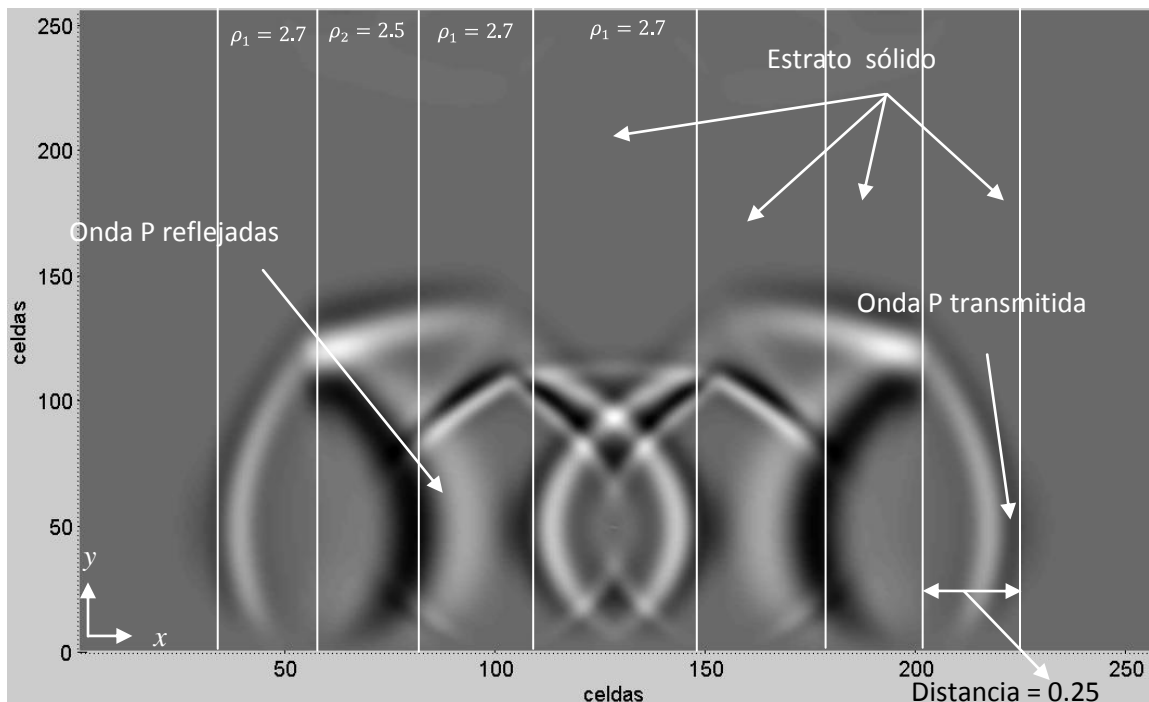
Figura 4.17. Propagación de las ondas P, en un multi-estrato sólido en una instantánea de un tiempo de 0.00058 segundos.
