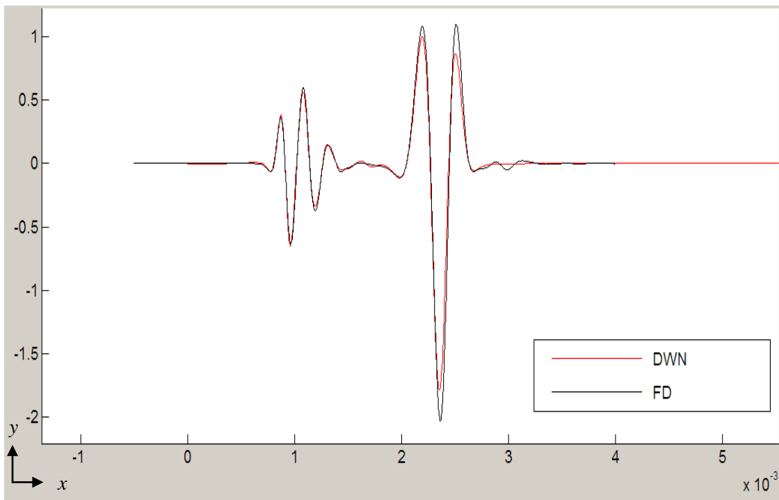
Figura 4.3. Representación del método diferencias finitas frente al método de ondas de discreta para diferentes valores.
