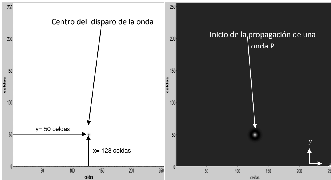
Figura 4.20. Inicio de una Propagación de la onda P en un estrato líquido, en una instantánea de un Tiempo de 0.000055 y 0.00013 segundos.
