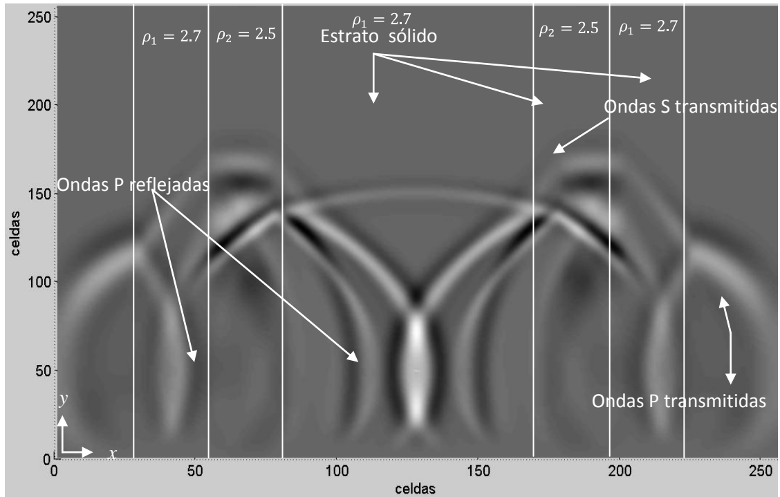
Figura 4.12. Propagación de ondas P y S en un medio estratificado sólido, en una instantánea de un tiempo de 0.00080 segundos.
