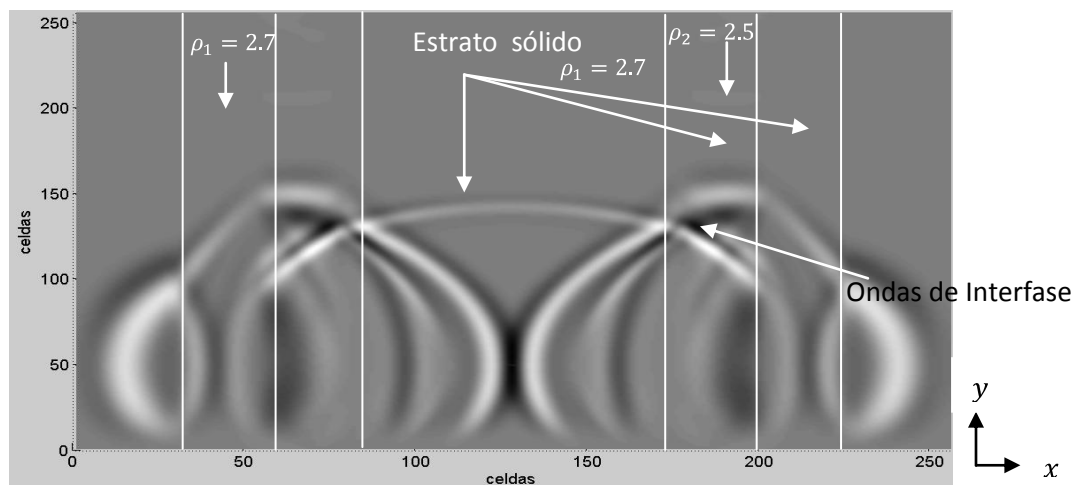
Figura 4.11. Propagación de ondas de Interfase, en un instante de tiempo 0.00074 segundos
