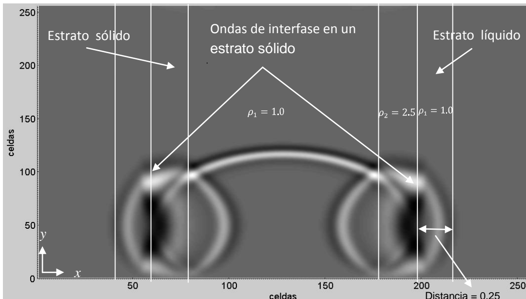
Figura 4.24. Propagación de las ondas de Interfase, en un medio líquido confinados con dos medios solidos, en un instante de un tiempo de 0.00058 segundos.
