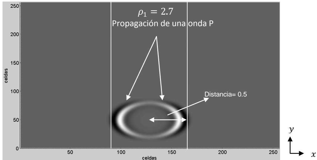
Figura 4.6. Propagación de una onda, en una instantánea de un tiempo de 0.00033 segundos.
