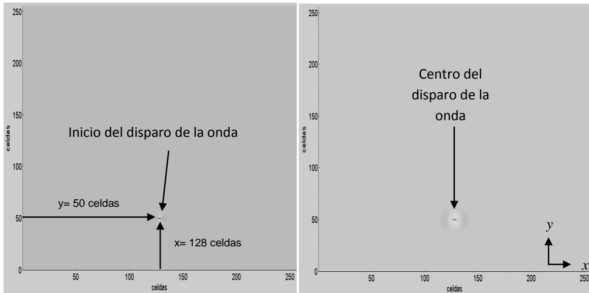
Figura 4.14. Inicio de la propagación de una onda P, en una instantánea de un tiempo 0.00013 y 0.00016 segundos
