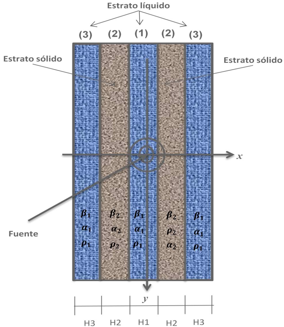
Figura 4.19. Sistemas de un medio estratificado líquido-sólido y simétrico, con distintas propiedades mecánicas.
