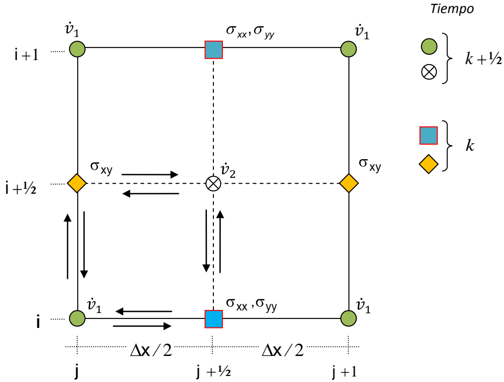
Figura 3.4. Esquema de malla alternada en espacio y tiempo.
