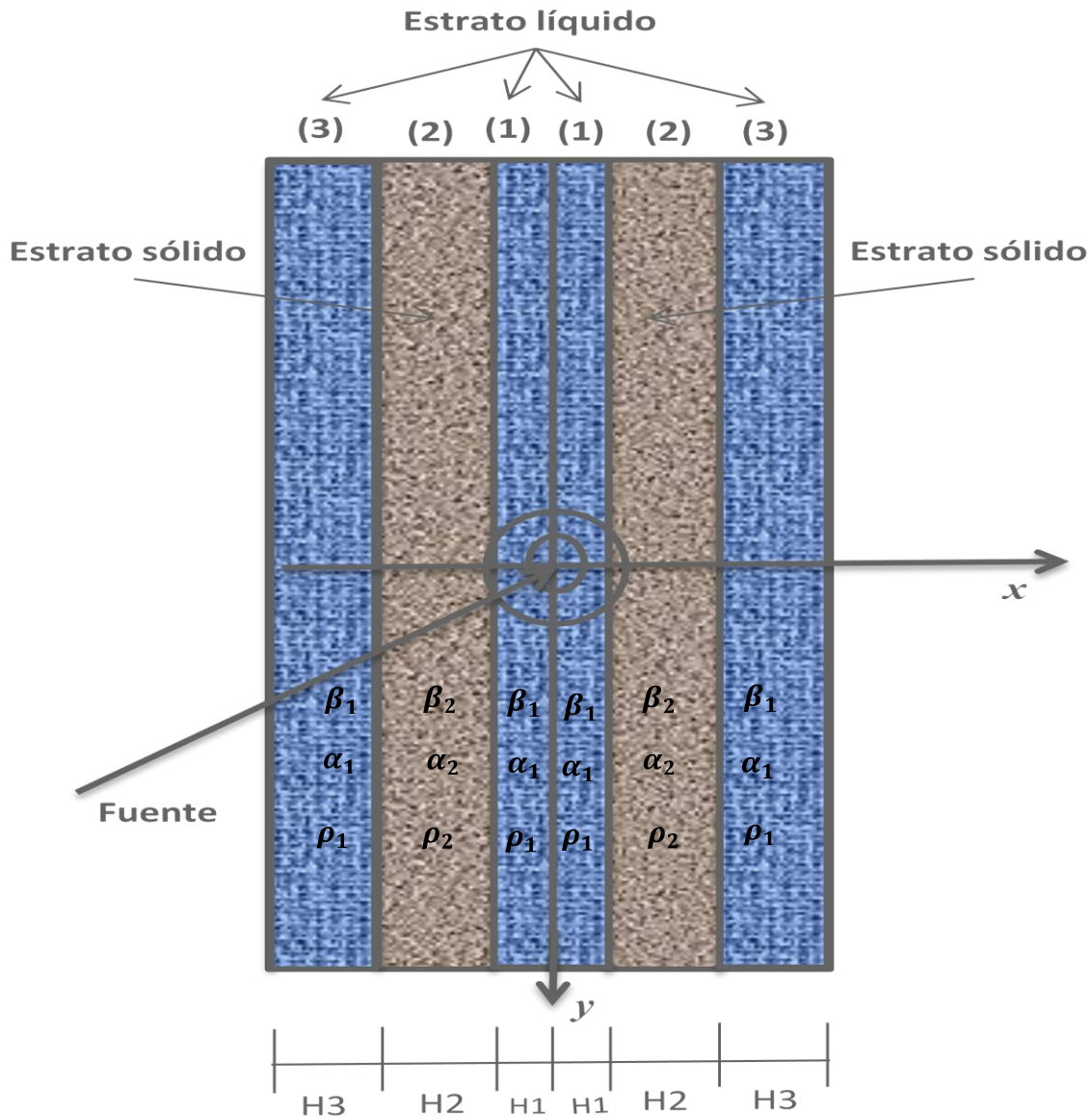
Figura 4.29. Sistemas de multi-estrato líquido-sólido y simétrico, con distintas propiedades mecánicas.
