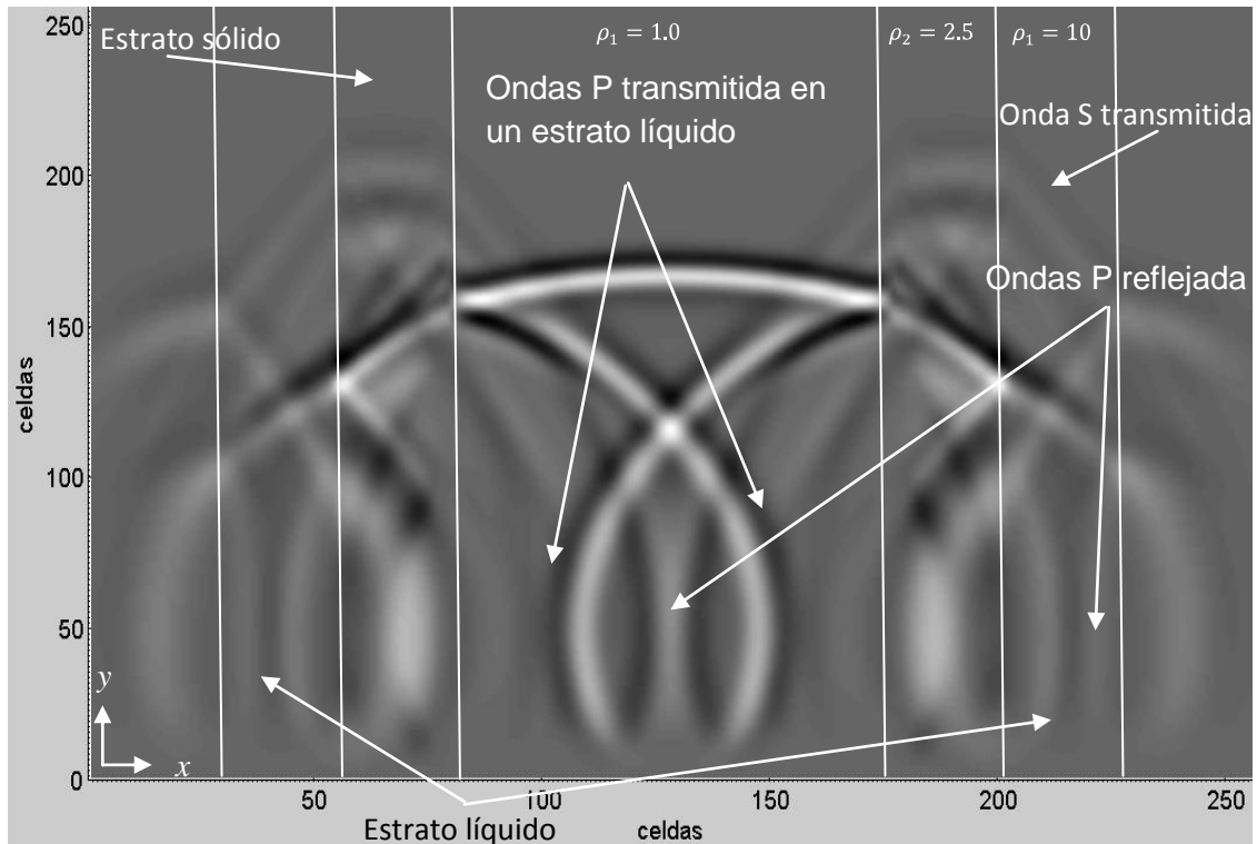
Figura 4.27. Propagación de las ondas P Transmitidas y Reflejadas en un multi-estrato Líquido-sólido, en una instantánea de un tiempo de 0.00091 segundos.
