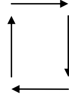
Fig. 3.3 (b). Distribución de fuerzas correspondiente a una explosión que genera una onda S
