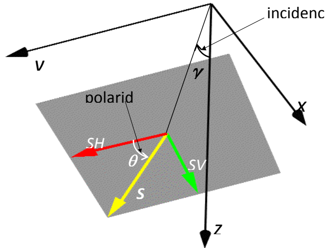
Fig. 1.3. La onda S y sus componentes SV y SH, el ángulo \gamma es el ángulo de incidencia y está definido en el plano x-z, el ángulo \theta queda comprendido entre la componente SH y la onda plana S
