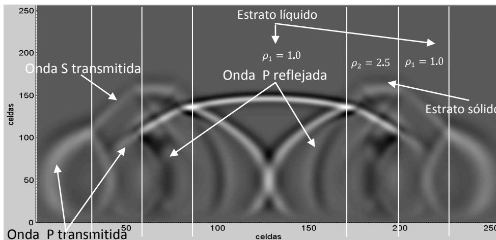
Figura 4.26. Propagación de ondas transmitidas y reflejadas en un multi-estrato líquido-sólido, en un instante de tiempo de 0.00077 segundos.
