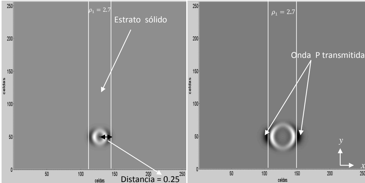
Figura 4.15. Propagación de una onda P transmitida, en una instantánea de un tiempo de 0.00019 y 0.00024 segundos.
