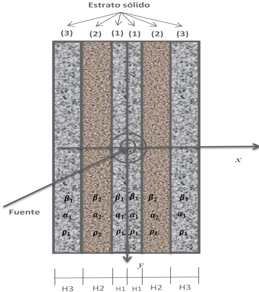
Figura 4.13. Sistemas de multi-estrato sólido y simétrico, con distintas propiedades mecánicas.
