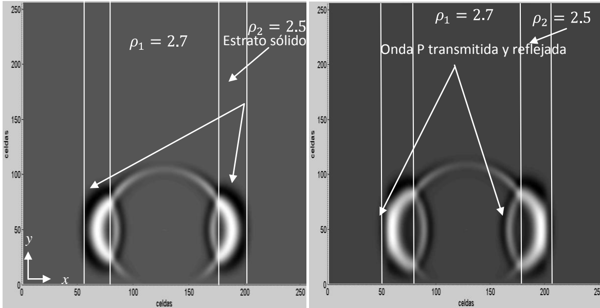
Figura 4.9. Propagación de ondas P transmitida y reflejada, en una instantánea de un tiempo de 0.00049 y 0.00052 segundos.
