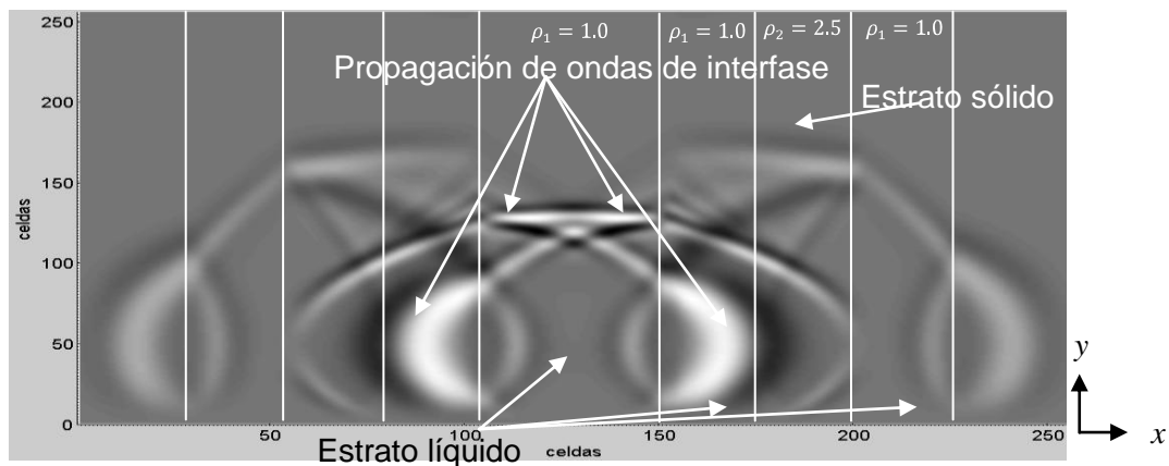
Figura 4.35. Propagación de las ondas de Interfase, en un multi-estrato líquido-sólido, en un instante de un tiempo de 0.00066 segundos.
