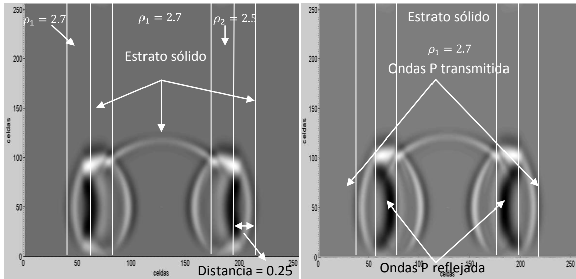
Figura 4.10. Propagación de una P transmitida y reflejada, en una instantánea de un tiempo de 0.00058 y 0.00061 segundos.
