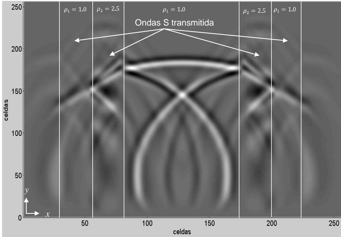
Figura 4.28. Propagación de las ondas S Transmitida en un multi-estrato líquido-sólido, con una instantánea de un tiempo de 0.0010 segundos.
