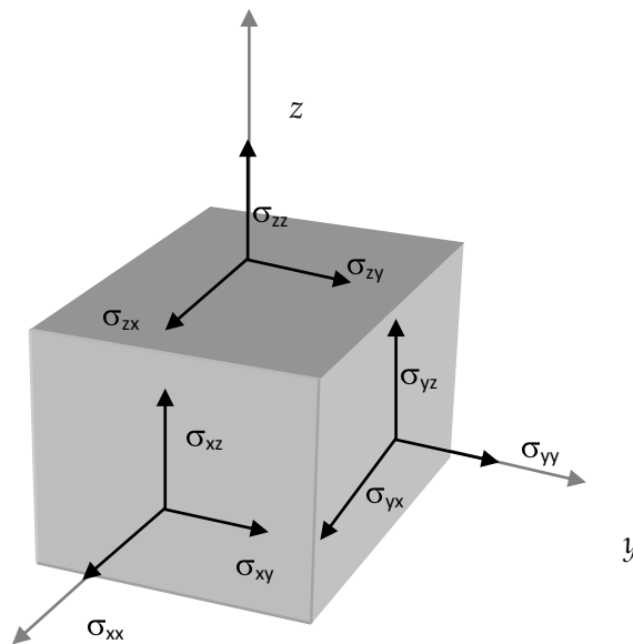
Fig. 2.2. Representación de esfuerzos en un volumen elemental. El primer subíndice indica la cara del paralelepípedo rectangular en la que actúa el esfuerzo y el segundo la dirección de dicho esfuerzo. Las caras indicadas son positivas y los esfuerzos representados tienen direcciones positivas. En las caras negativas, los esfuerzos positivos tendrán direcciones contrarias.
