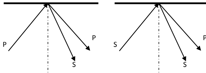
Figura 3.10. Detalle de las reflexiones en la superficie libre, tras la incidencia de onda P y S.
