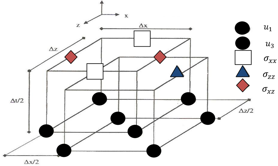
Figura.3.8. Discretización del medio con una malla alternada para el problema P-SV.
