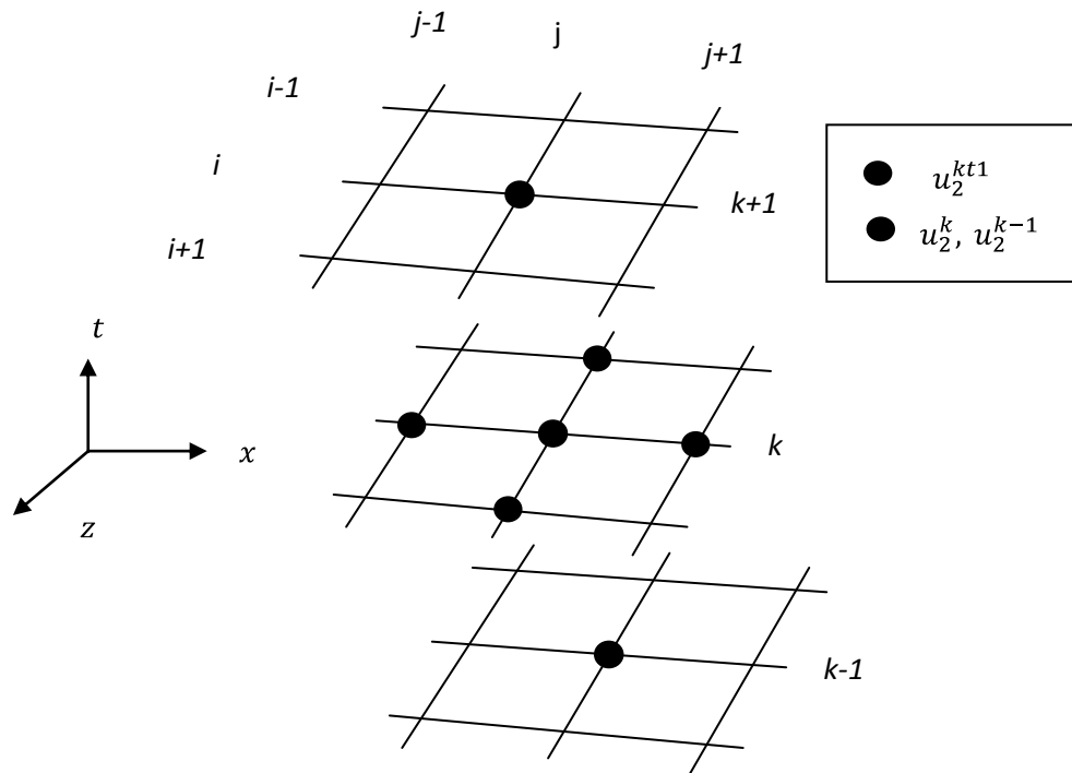
Figura 3.5. Esquema de discretización para el caso SH en 2D mediante el método de diferencias finitas.
