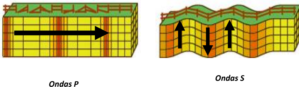
Fig. 1.2. Ondas de cuerpo.
