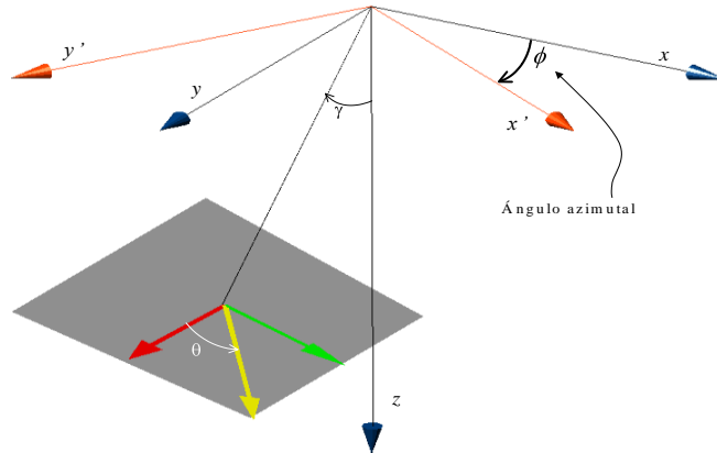
Fig. 1.4. Definición del ángulo azimutal.
