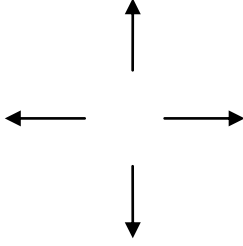
Fig. 3.3 (a). Distribución de fuerzas correspondiente a una explosión que genera una onda P
