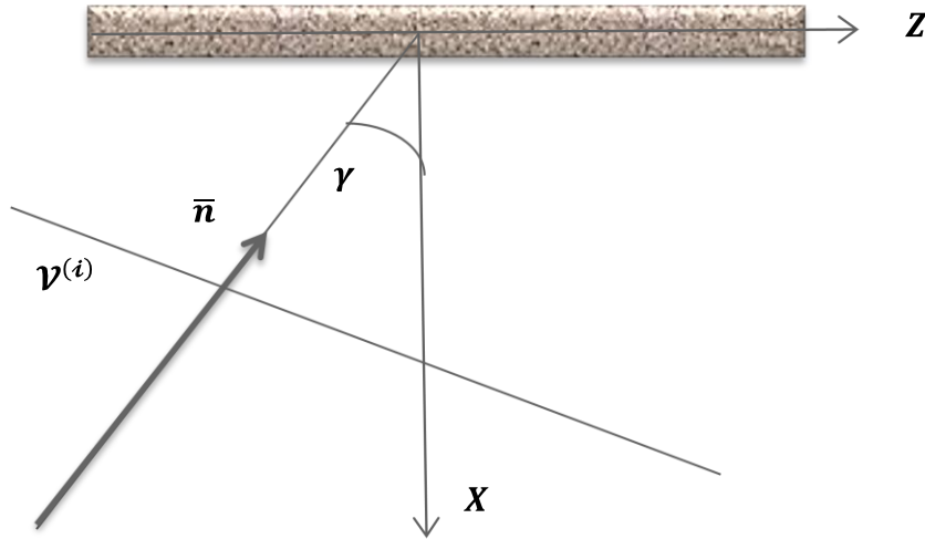
Figura 2.3. Onda SH incidente
