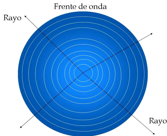
Fig. 1.1 Frentes de onda propagándose hacia fuera. Las líneas perpendiculares a los frentes de onda se denominan Rayos, e indican la trayectoria de propagación.
