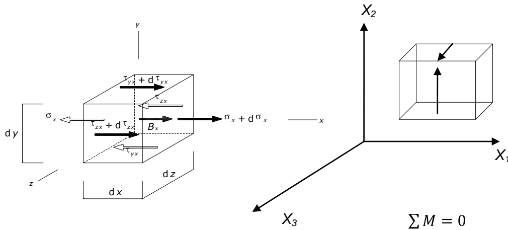
Figura 2.3. Representación de la Ecuación de Movimiento
