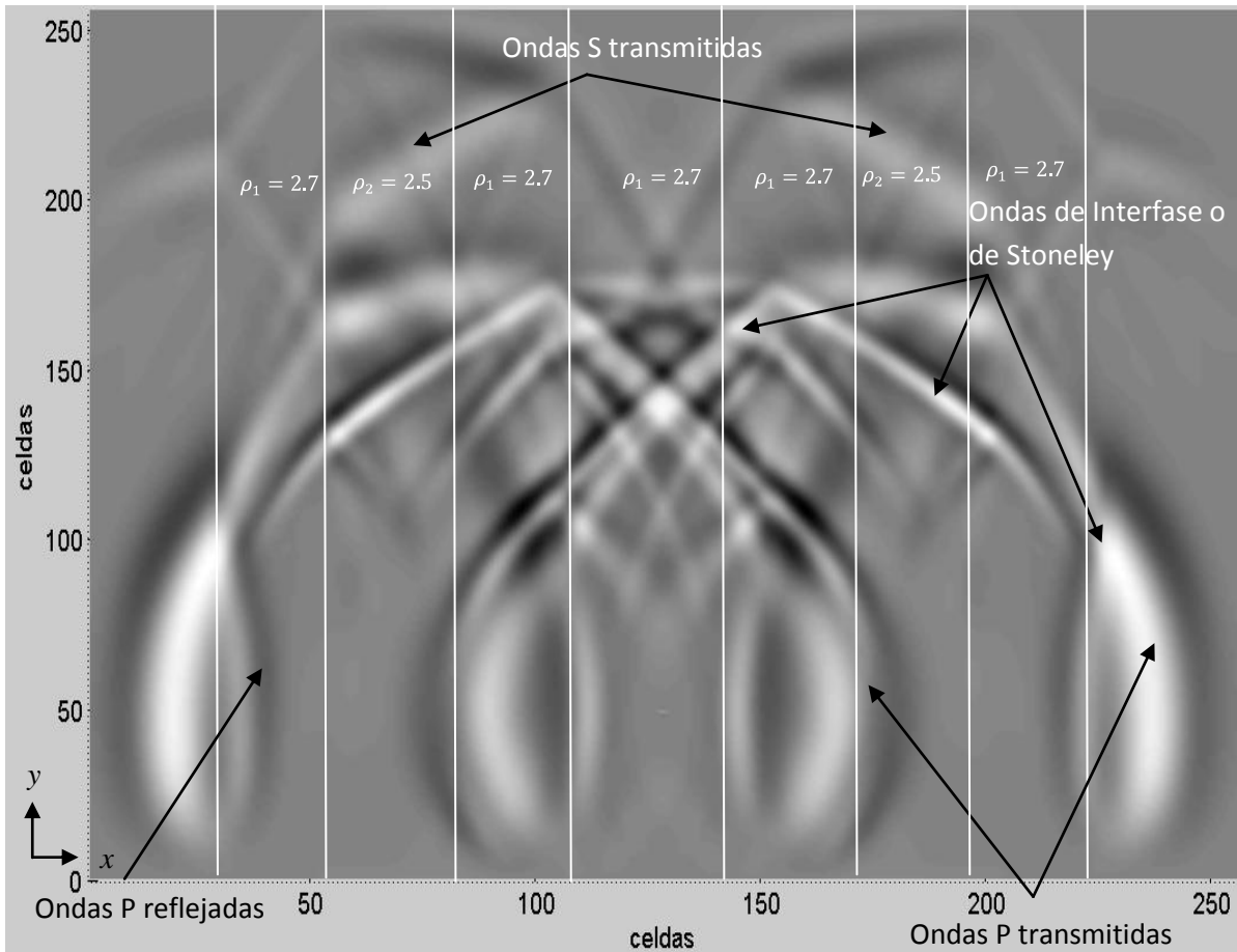
Figura 4.18. Propagación de ondas de Interfase o Stoneley en un multi-estrato sólido en una instantánea de un tiempo de 0.00097 segundos.
