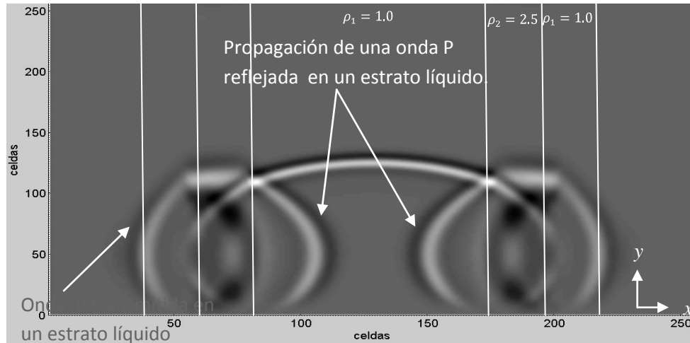
Figura 4.25. Propagación de las ondas P reflejadas y transmitidas, en una instantánea de un tiempo de 0.00063 segundos.
