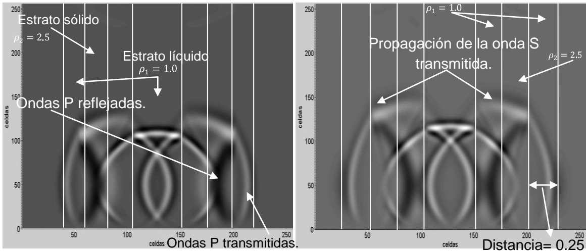
Figura 4.34. Propagación de las ondas P y S transmitida en un multi-estrato líquido-sólido, con una instantánea de un tiempo de 0.00052 y 0.00058 segundos.
