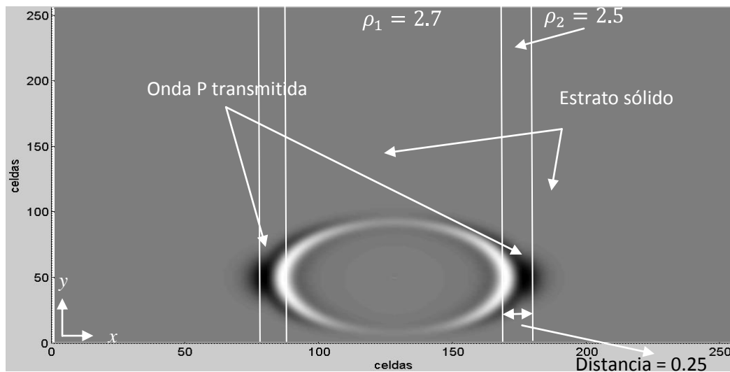
Figura 4.8. Propagación de una onda P transmitida, en un instante de un tiempo de 0.00041 segundos.
