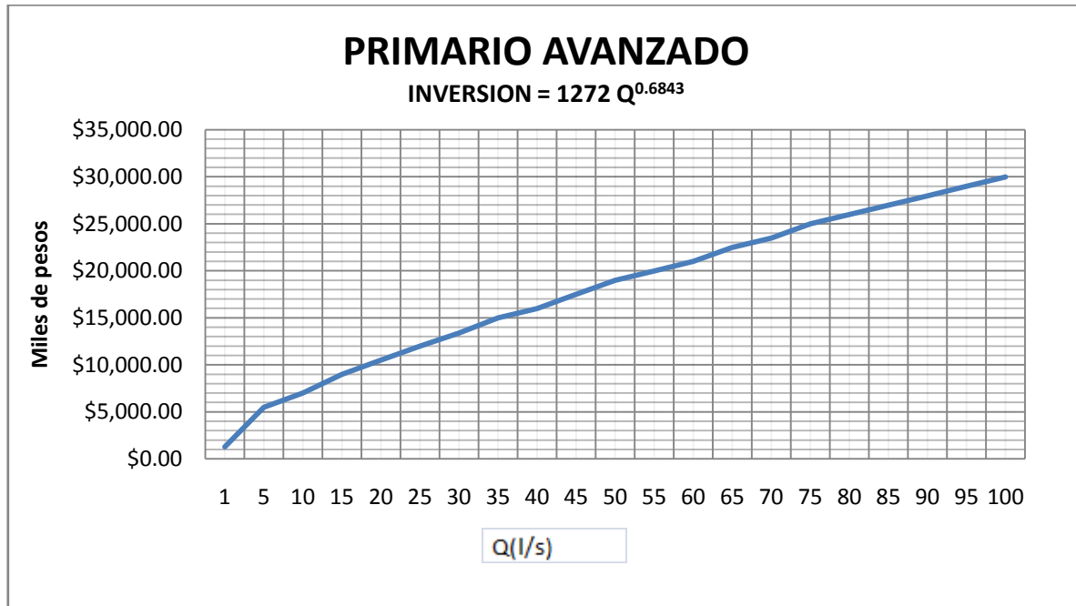
Grafica # 3.- Grafica de costo de inversión de tratamiento Primario Avanzado. Obtención: Morales, G. Servín, C. Montesillo, J. Escalante V. Rivas A. (2002). Aplicación de Costos Índice de Plantas de Tratamiento de Aguas Residuales . IMTA. México. Pág. 12.
