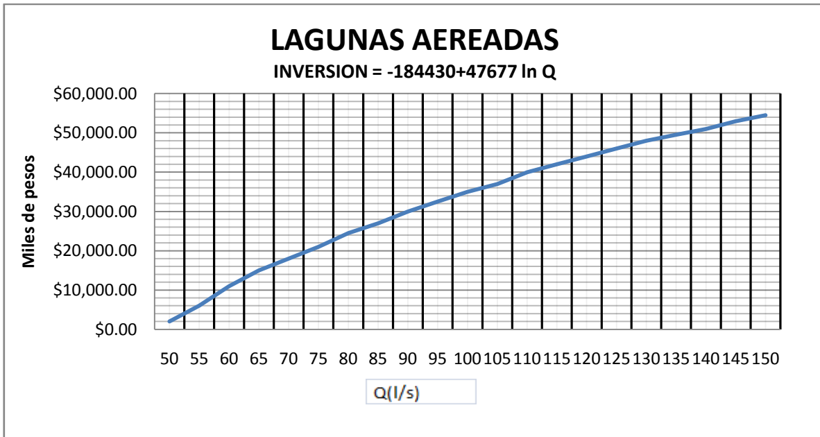
Grafica # 6.- Grafica de costo de inversión de tratamiento Lagunas Aereadas. Obtención: Morales, G. Servín, C. Montesillo, J. Escalante V. Rivas A. (2002). Aplicación de Costos Índice de Plantas de Tratamiento de Aguas Residuales . IMTA. México. Pág. 18.
