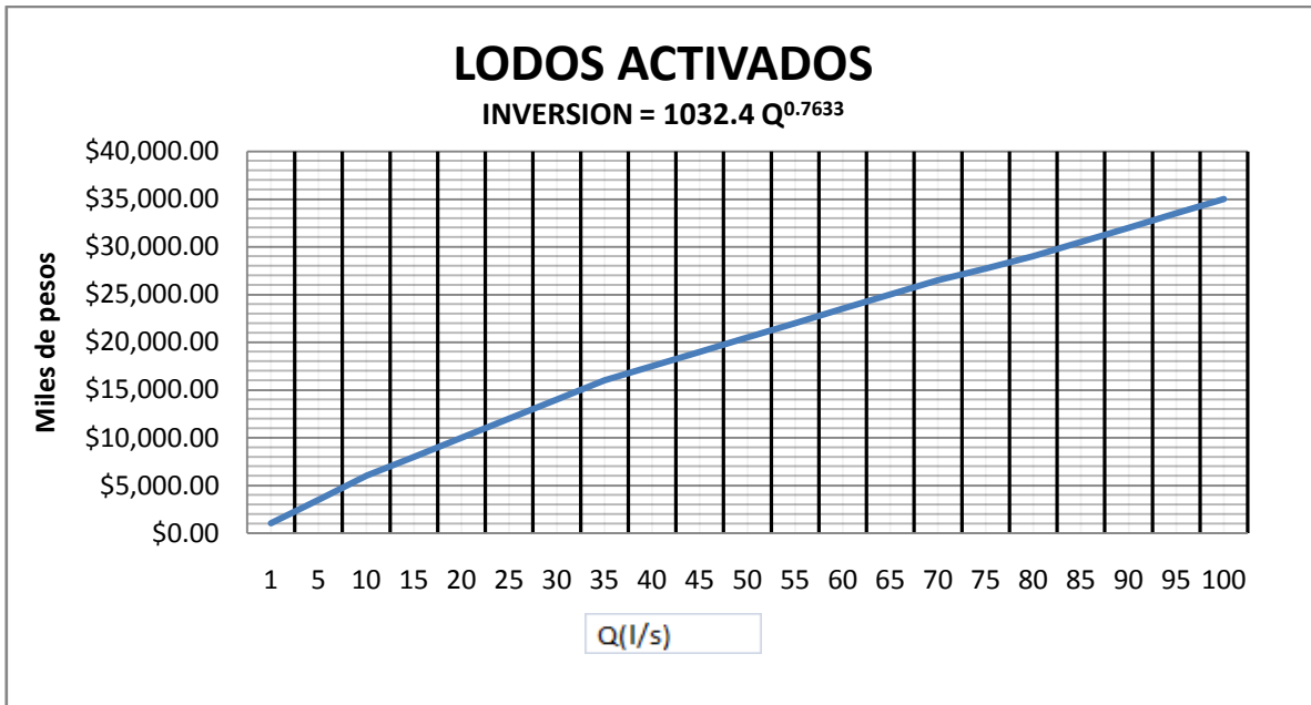
Grafica # 4.- Grafica de costo de inversión de tratamiento de Lodos Activados. Obtención: Morales, G. Servín, C. Montesillo, J. Escalante V. Rivas A. (2002). Aplicación de Costos Índice de Plantas de Tratamiento de Aguas Residuales . IMTA. México. Pág. 14.
