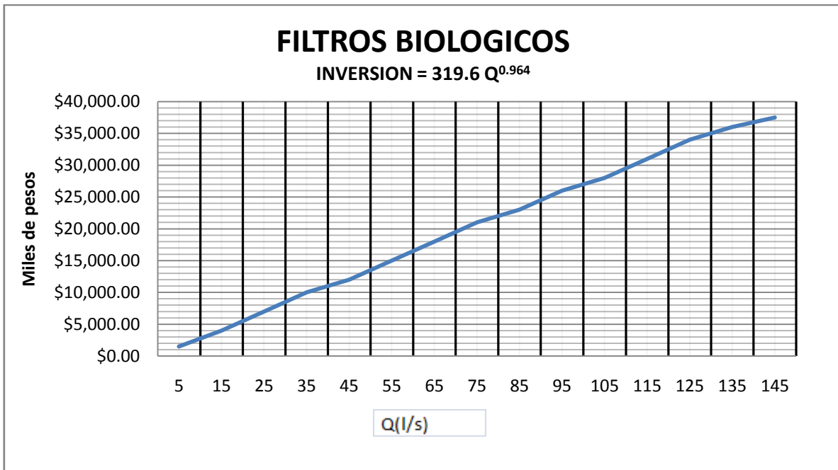
Grafica # 5.- Grafica de costo de inversión de tratamiento de Filtros Biológicos. Obtención: Morales, G. Servín, C. Montesillo, J. Escalante V. Rivas A. (2002). Aplicación de Costos Índice de Plantas de Tratamiento de Aguas Residuales . IMTA. México. Pág. 16.
