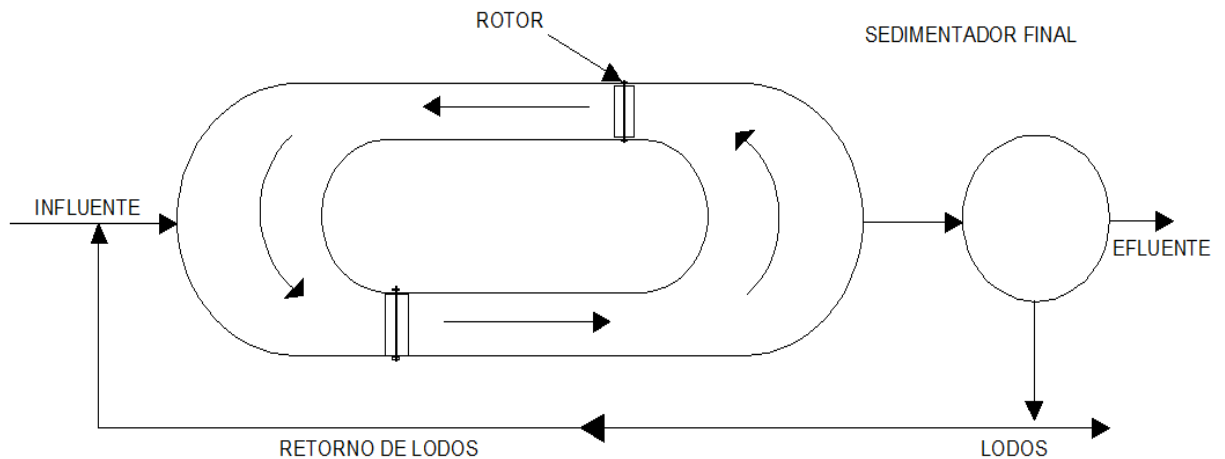
Esquema #5 Proceso de tratamiento por medio de Zanjas de Oxidación. Realizado en AutoCAD 2009 Elaborado con datos obtenidos de: CONAGUA. (1994). Sistemas alternativos de tratamiento de aguas residuales y lodos producidos . Pág. 264.
