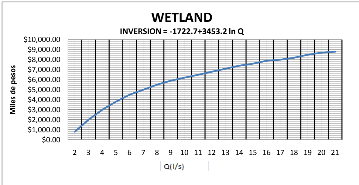
Grafica # 8.- Grafica de costo de inversión de tratamiento Wetland. Obtención: Morales, G. Servín, C. Montesillo, J. Escalante V. Rivas A. (2002). Aplicación de Costos Índice de Plantas de Tratamiento de Aguas Residuales . IMTA. México. Pág. 22.
