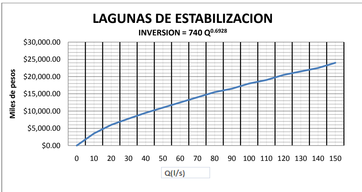
Grafica # 7.- Grafica de costo de inversión de tratamiento Lagunas de Estabilización. Obtención: Morales, G. Servín, C. Montesillo, J. Escalante V. Rivas A. (2002). Aplicación de Costos Índice de Plantas de Tratamiento de Aguas Residuales . IMTA. México. Pág. 20.
