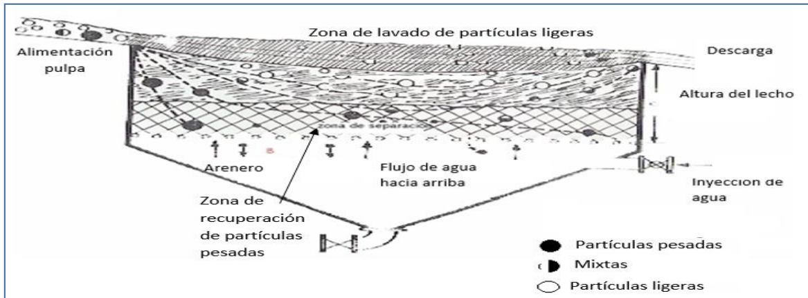
Figura 15. Pulsadora básica
