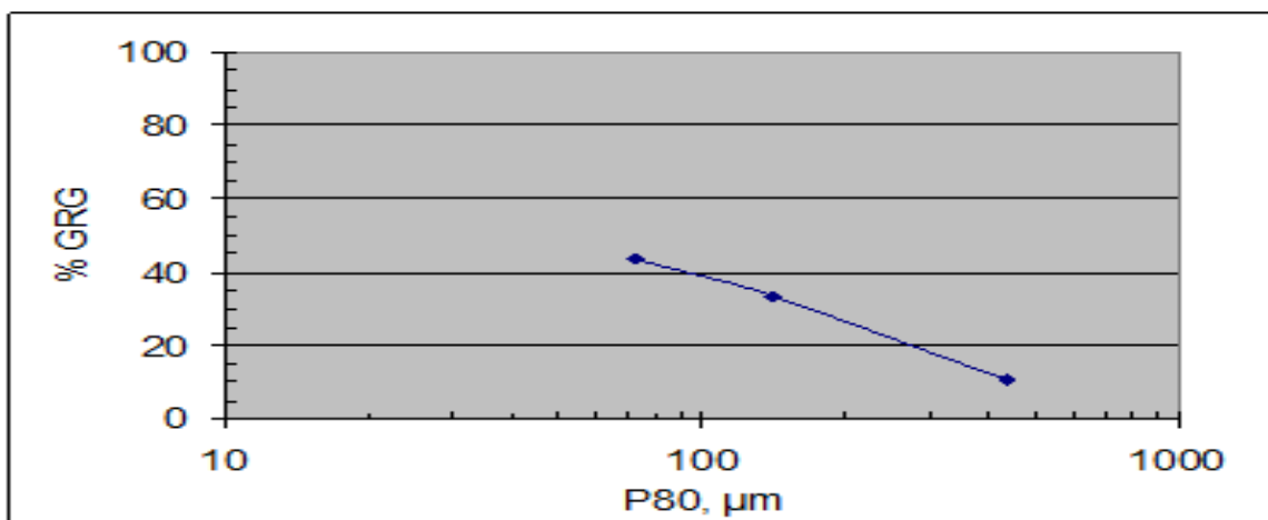
Fig. 7. % de GRG como función de la molienda P80
