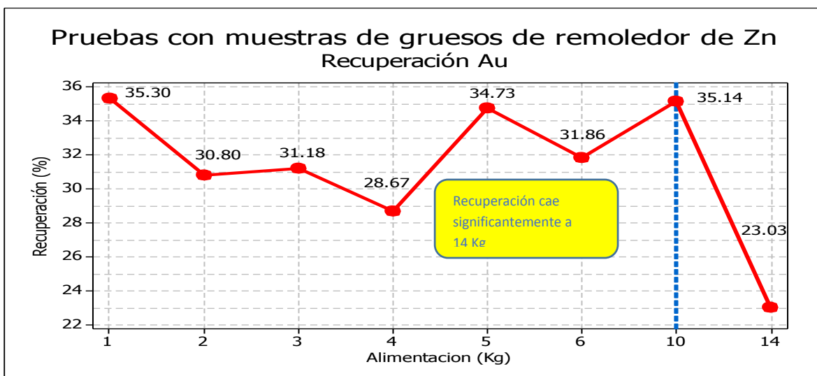
Figura 48. Recuperación de Au con gruesos de remolador de zinc variando la alimentación
