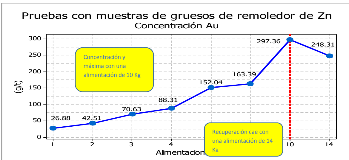
Figura 47. Concentración de Au con gruesos de remolador de zinc variando la alimentación.
