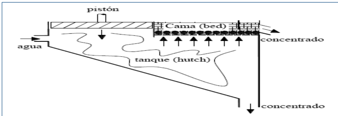
Figura 16. Pulsadora Harz.
