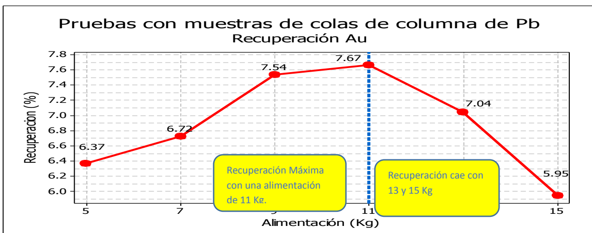
Figura 52. Recuperación de Au con colas de columna de plomo variando alimentación.
