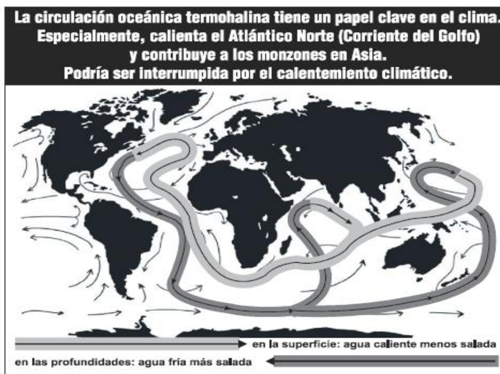
Figura 3.3 la circulación termohalina
