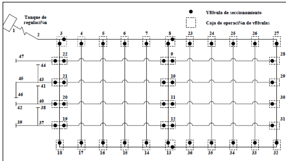
Figura 2. 11 Red secundaria en bloques
