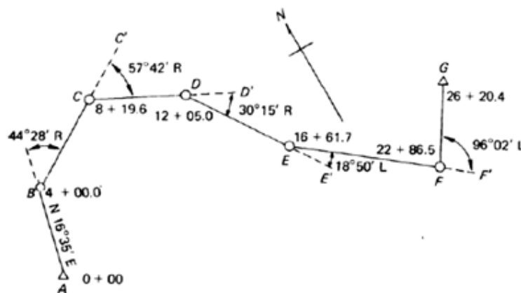
Figura 1. 14 Poligonal abierta con ángulos exteriores
