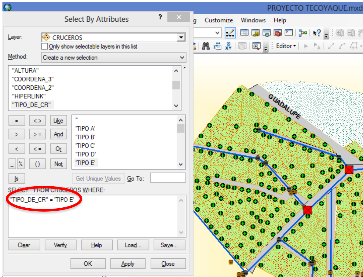
Figura 4.51 Selección de tipo de cruceo.
