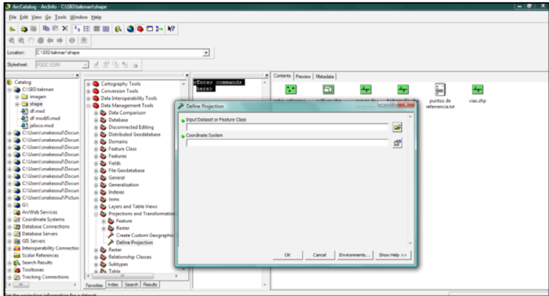
Figura 4.19 Vista Definir Proyección
