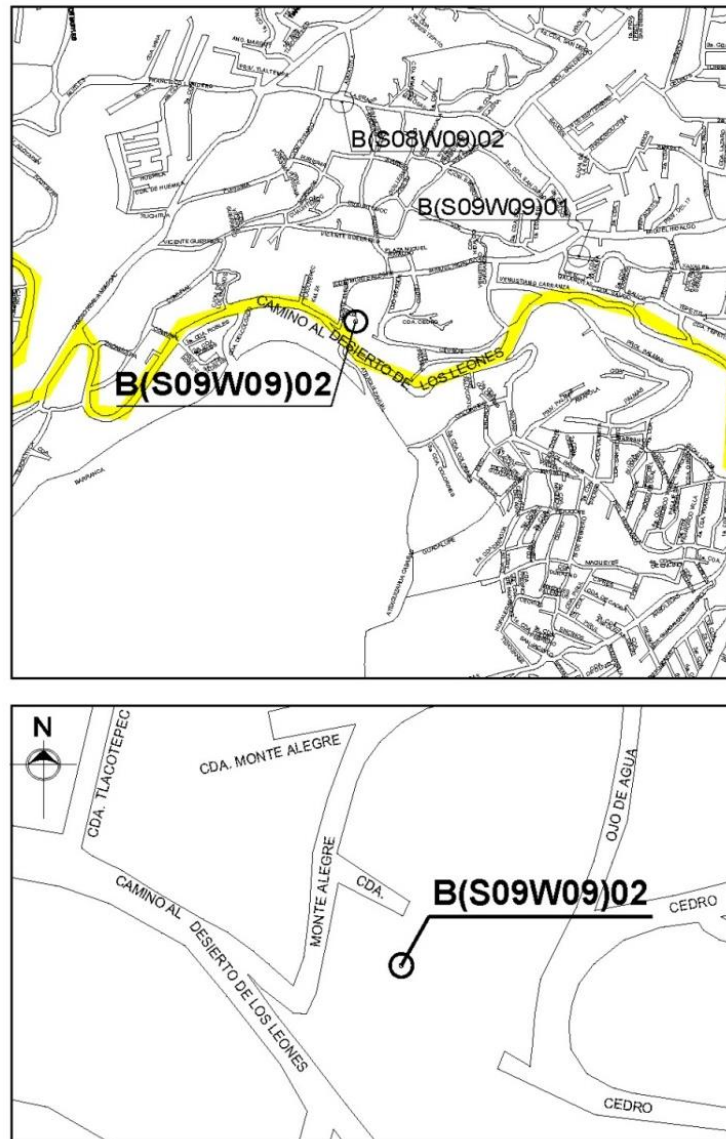
Figura 4.9 Croquis de localización del Banco de Nivel Oficial B(S09W09)02 (Copias proporcionadas por el SACMEX).
