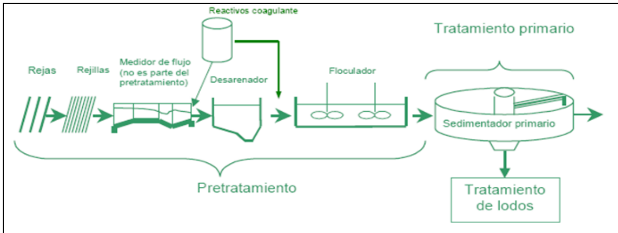
Figura 2. 22 Planta típica de Tratamiento de aguas residuales Tipo Primario
