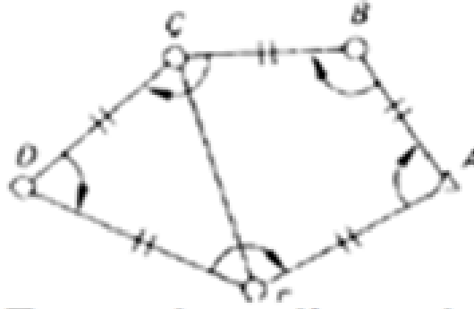
Figura 1. 13 Poligonal cerrada con ángulos interiores
