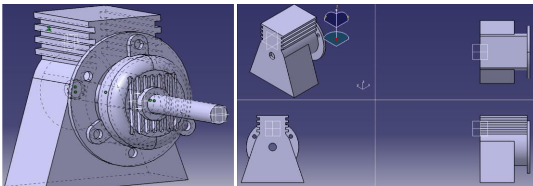
Figura 39. Vistas del dibujo mecánico del motor acoplado para el soplador (realizado en Catia V5)
