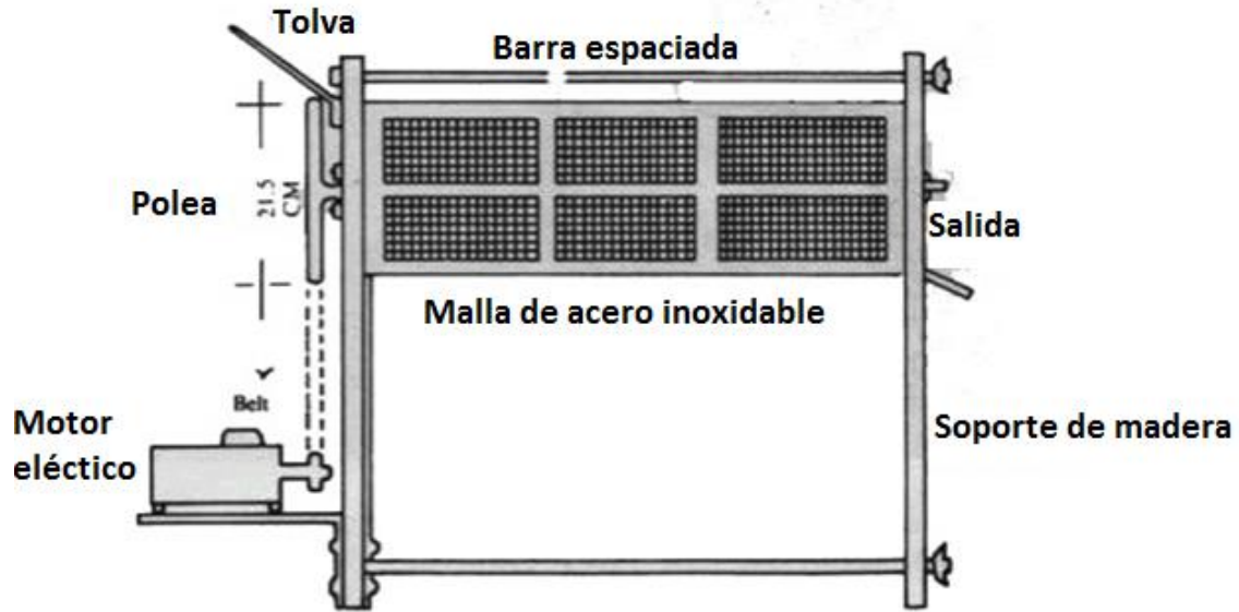
Figura 3. Mecanismo de mallas rotatorias
