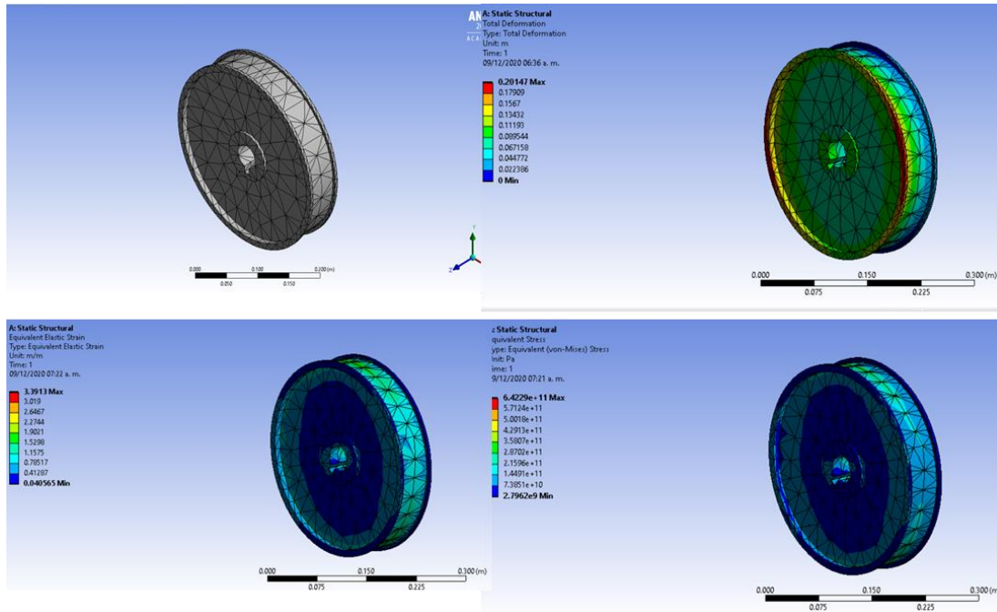
Figura 49. Mallado del rodetete dinámico y resultados de la simulación (Realizado en ANSYS Workbench 2020 R2)
