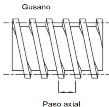
Figura 27. Nomenclatura general del tornillo sin fin (tomado de ANSI/ AGMA 6022)
