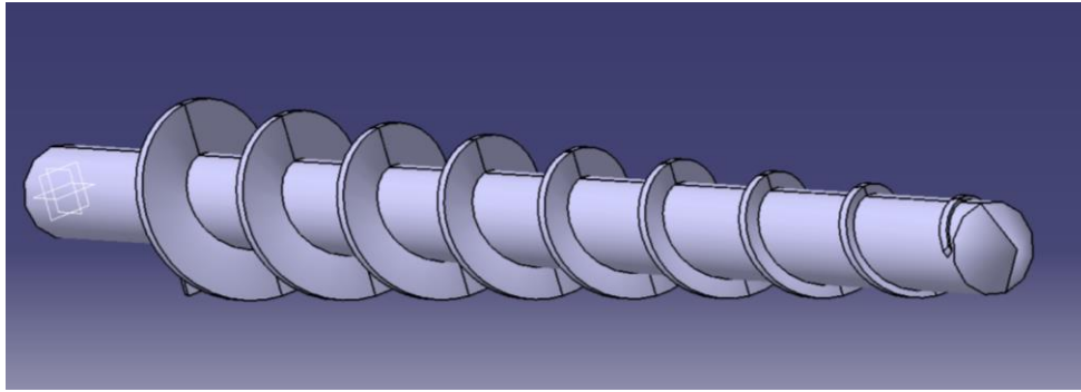
Figura 40. Vista isométrica del dibujo mecánico del tornillo sin fin para la extracción de aceite (realizado en Catia V5)
