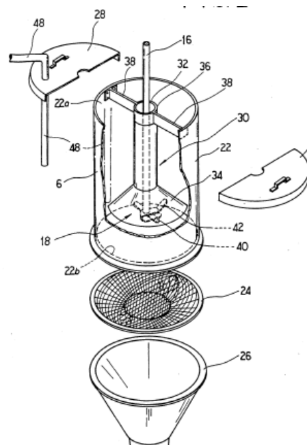
Figura 4. Triturador de semillas por tolvas
