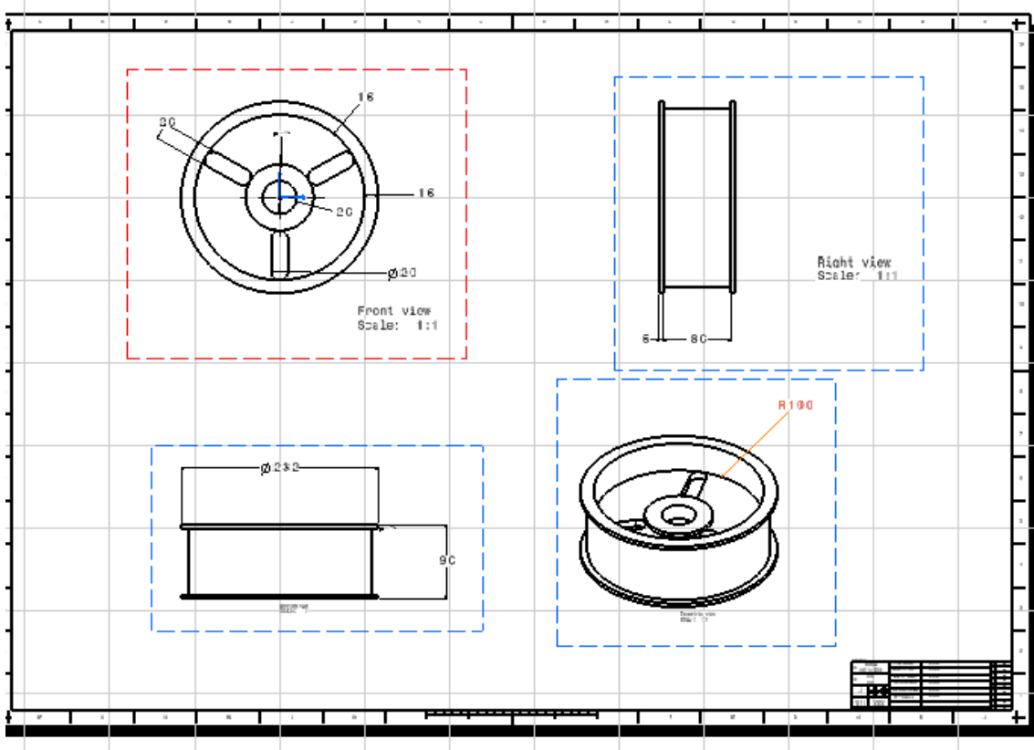
Figura 34. Plano mecánico de rodete compresor estático (ASME US Standard)
