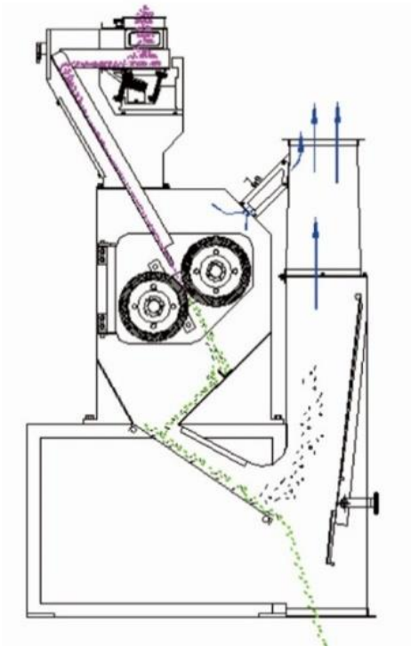
Figura 6. Mecanismo de rodetes giratorios para compresión de semillas
