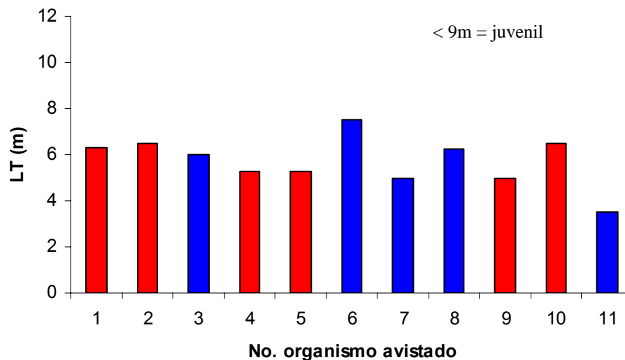
Figura 8. Longitudes totales (LT) de cada uno de los tiburones ballena avistados en la localidad de Bahía de los Ángeles durante octubre de 2004 (barras rojas= hembras, barras azules=machos).
