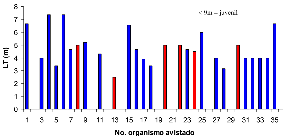
Figura 9. Longitudes totales (LT) de cada uno de los tiburones ballena avistados en la localidad de Bahía de La Paz durante octubre del año 2004 (barras rojas= hembras, barras azules=machos, espacio libres en eje x = sexo y longitud no registrada).
