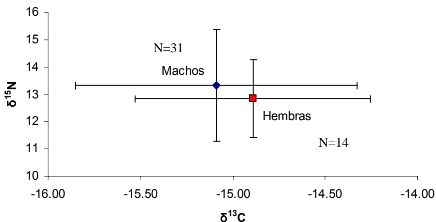
Figura 20. Medias y desviaciones estándar de los isótopos estables de \delta^{13}\text{C} y \delta^{15}\text{N} de machos y hembras. (BLA y BLP)
