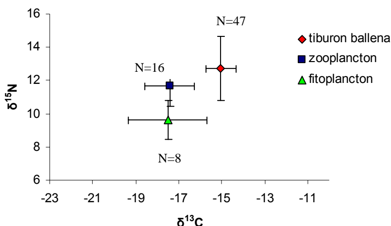
Figura 25. Medias y desviaciones estándar de los isótopos estables de \delta^{13}\text{C} y \delta^{15}\text{N} de tejido de tiburón ballena (depredador) y de plancton (presas), para el área de BLP
