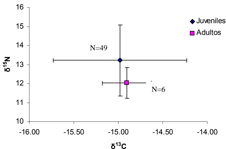
Figura 22. Medias y desviaciones estándar de los isótopos estables de \delta^{13}\text{C} y \delta^{15}\text{N} entre tiburones ballena juveniles (BLA y BLP) y adultos (BG).
