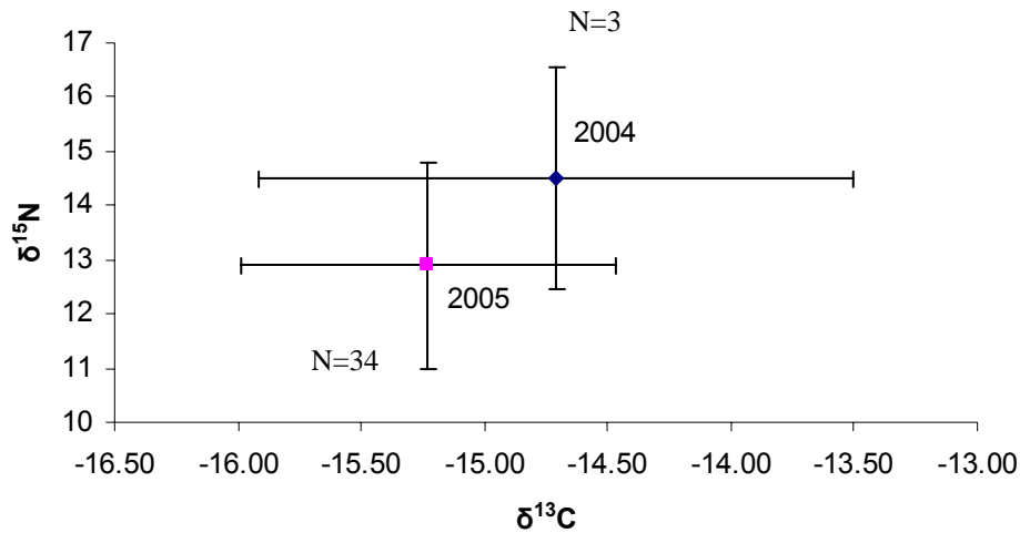
Figura 23. Medias y desviaciones estándar de los isótopos estables de \delta^{13}\text{C} y \delta^{15}\text{N} durante los años de estudio en BLP (2004 y 2005)
