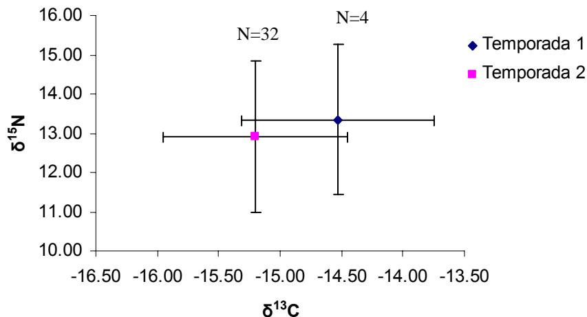
Figura 24. Medias y desviaciones estándar de los isótopos estables de \delta^{13}\text{C} y \delta^{15}\text{N} durante la primera temporada (abril a mayo) y la segunda temporada (septiembre a diciembre) en BLP.
