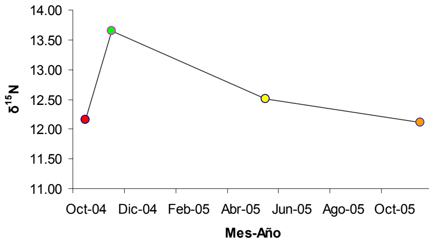
Figura 27. Valores de \delta^{15}\text{N} de un mismo tiburón muestreado en las localidades de BLA y BLP para distintos meses y año.
